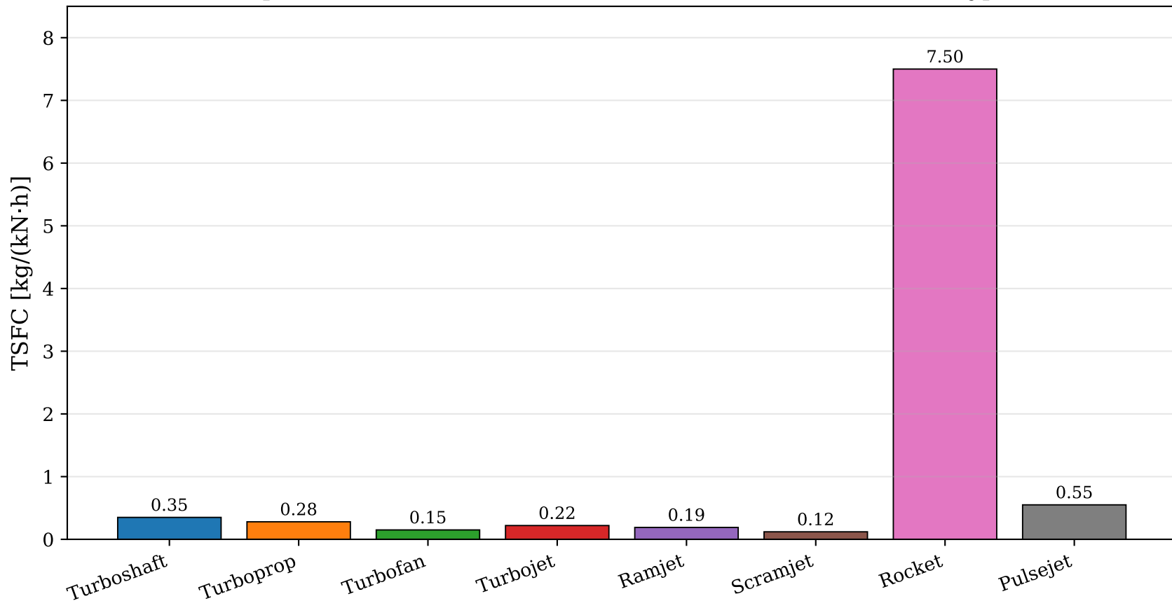
Spezifischer Kraftstoffverbrauch (TSFC) nach Triebwerkstyp
