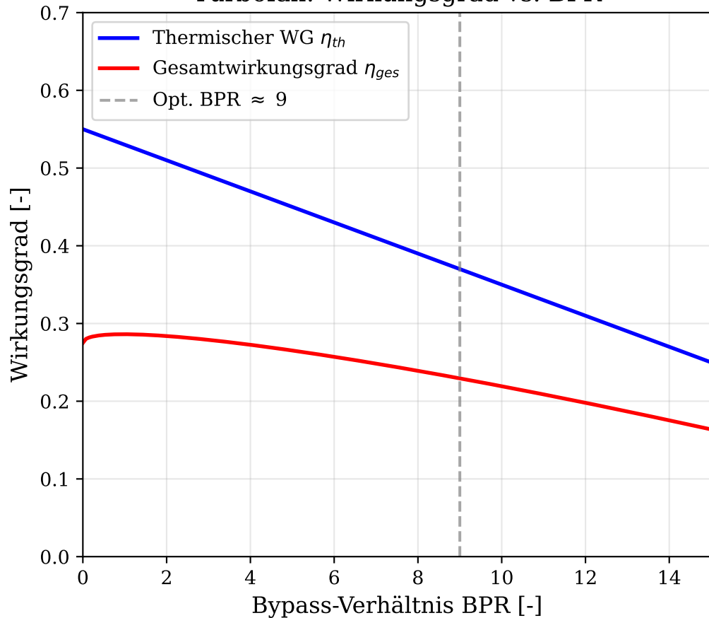
Turbofan: Wirkungsgrad vs. BPR
