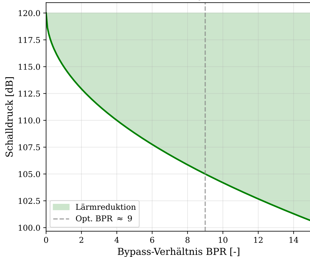
Turbofan: Lärmpegel vs. BPR
