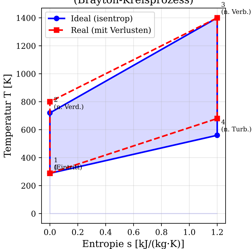
T-s Diagramm (Brayton-Kreisprozess)
