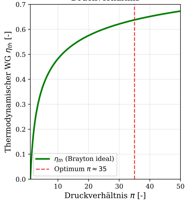
Wirkungsgrad vs. Druckverhältnis
