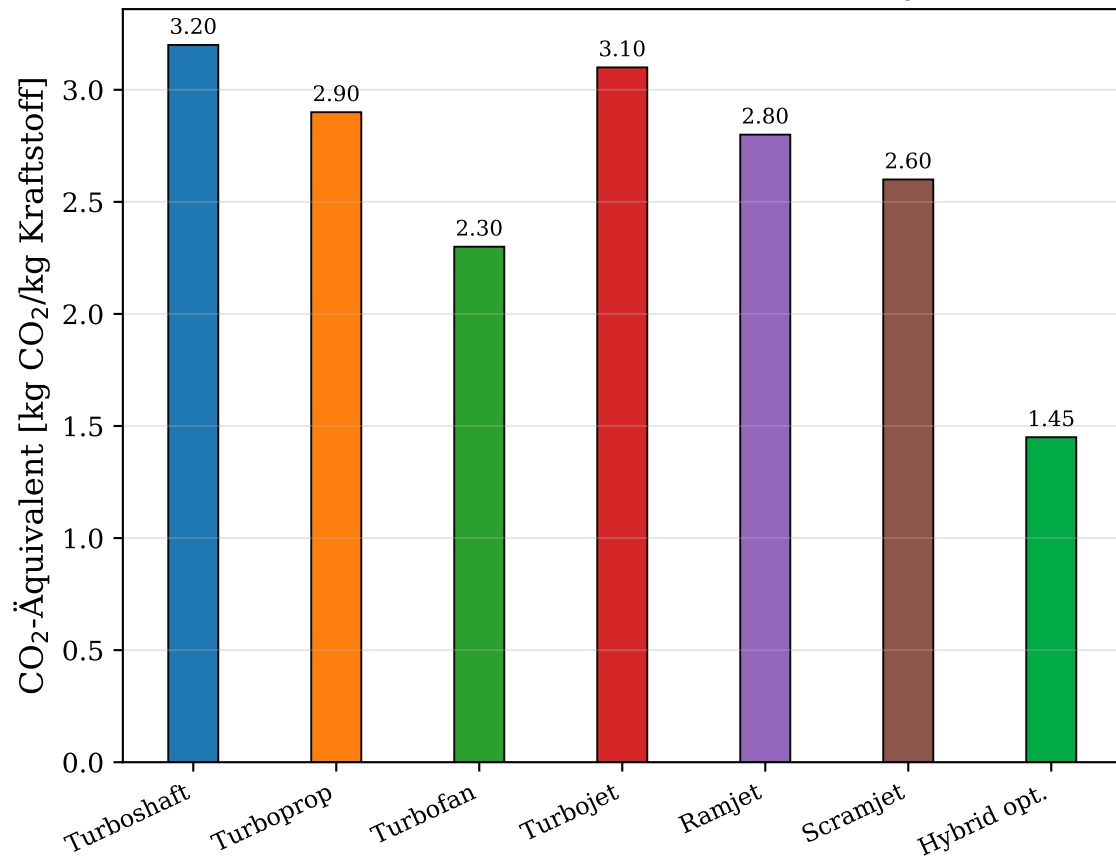
CO 2 -Emissionen nach Triebwerkstyp
