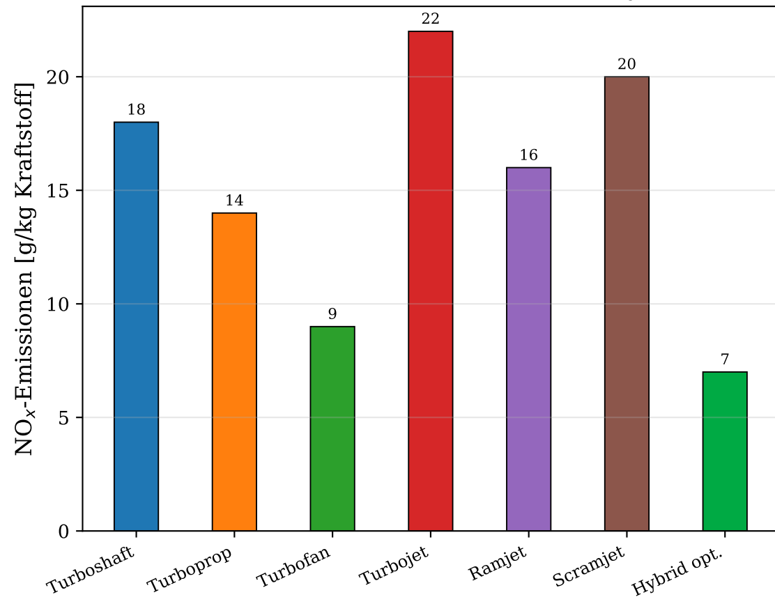
NO x -Emissionen nach Triebwerkstyp
