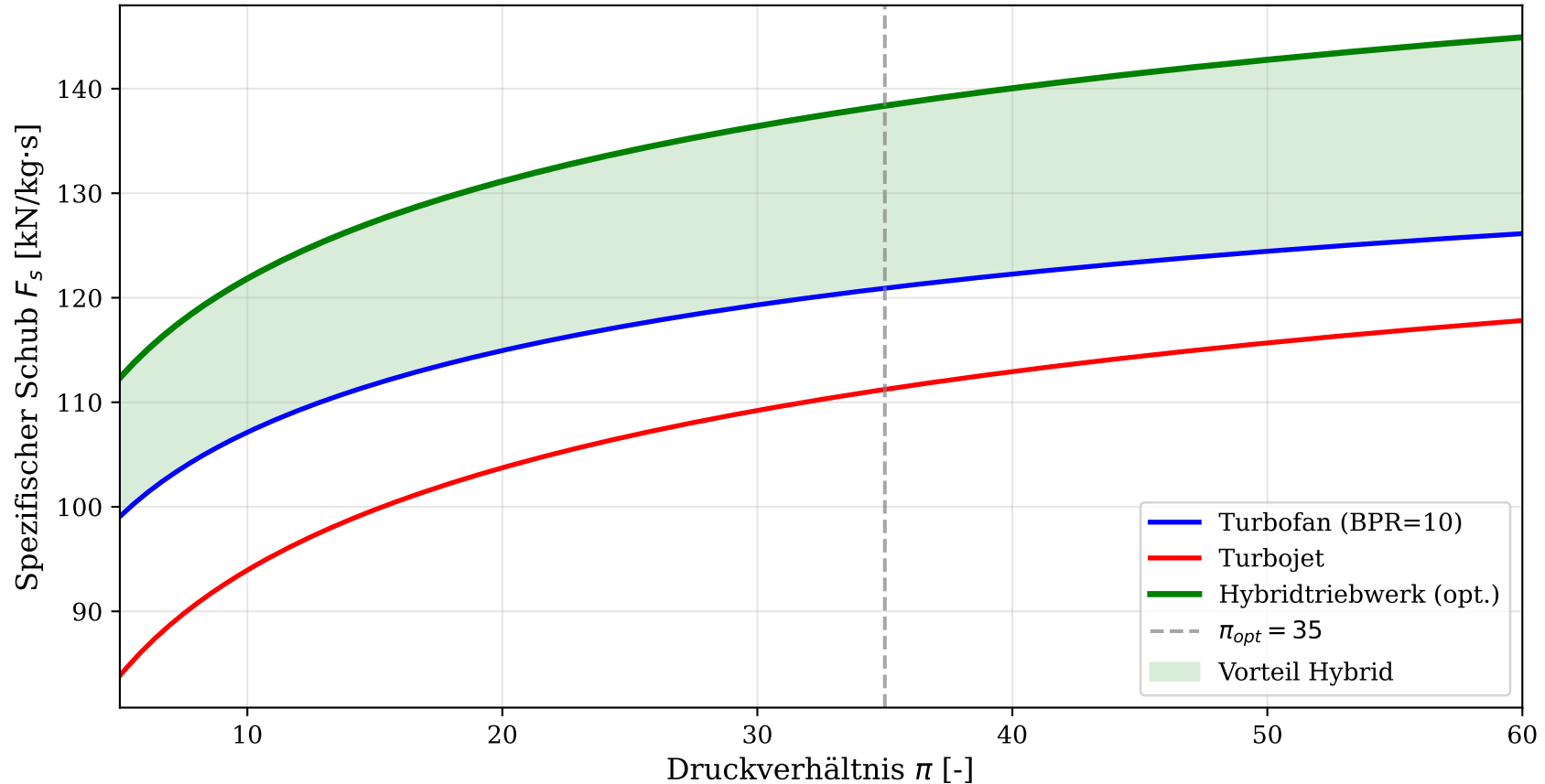
Spezifischer Schub in Abhängigkeit des Druckverhältnisses
