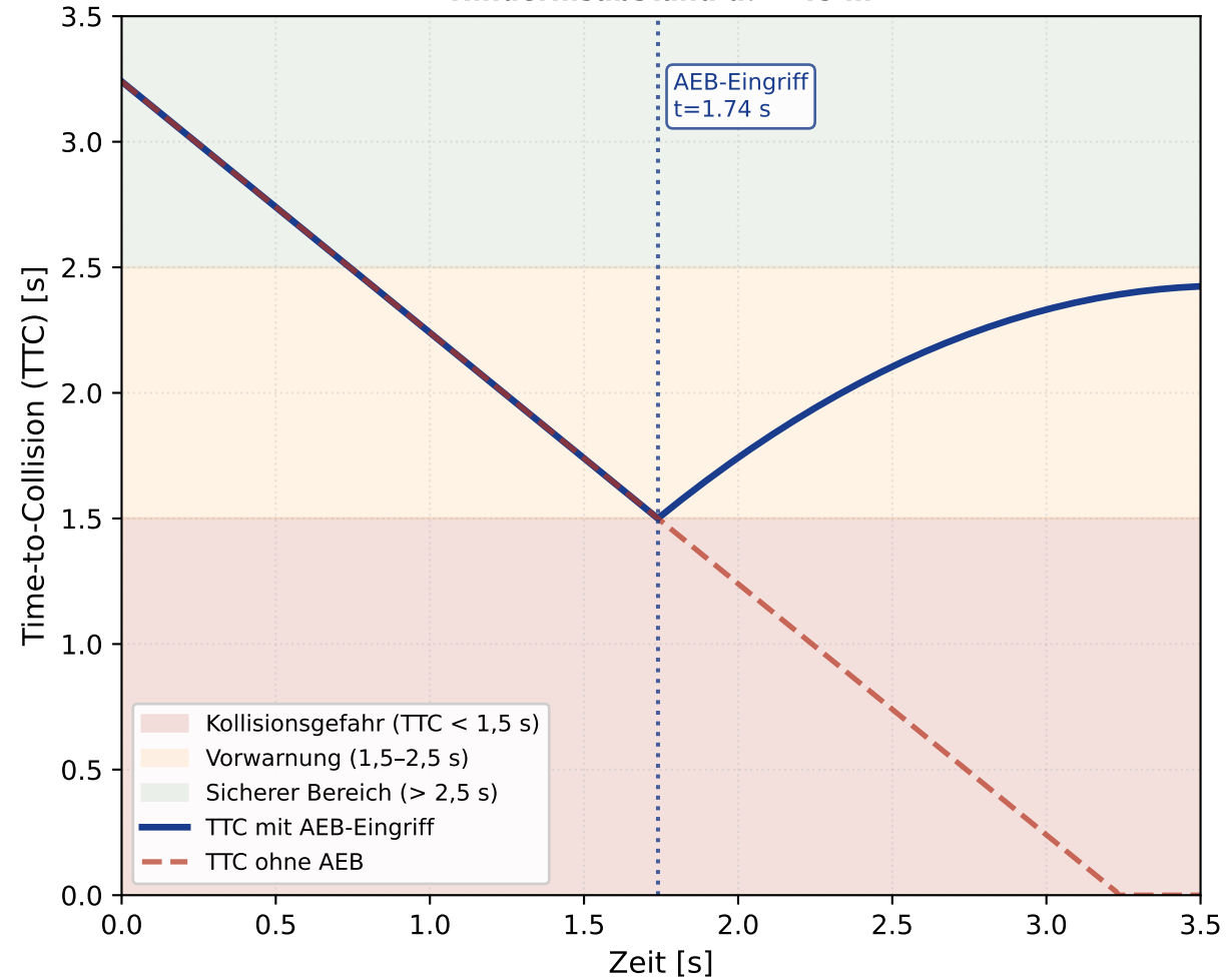
(b) TTC-Verlauf: AEB-Eingriff bei 50 km/h Hindernisabstand d_0 = 45 m
