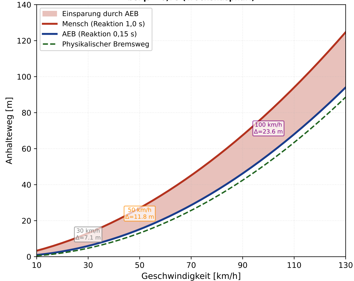
(a) Anhalteweg: Mensch vs. AEB bei \mu = 0,75 (Trockenasphalt)
