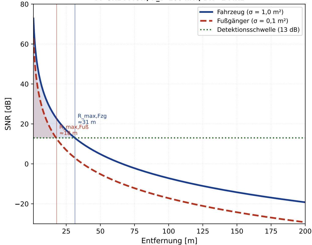
(a) Radargleichung: SNR vs. Entfernung 77 GHz FMCW, P_t=100 mW, BW=1 MHz
