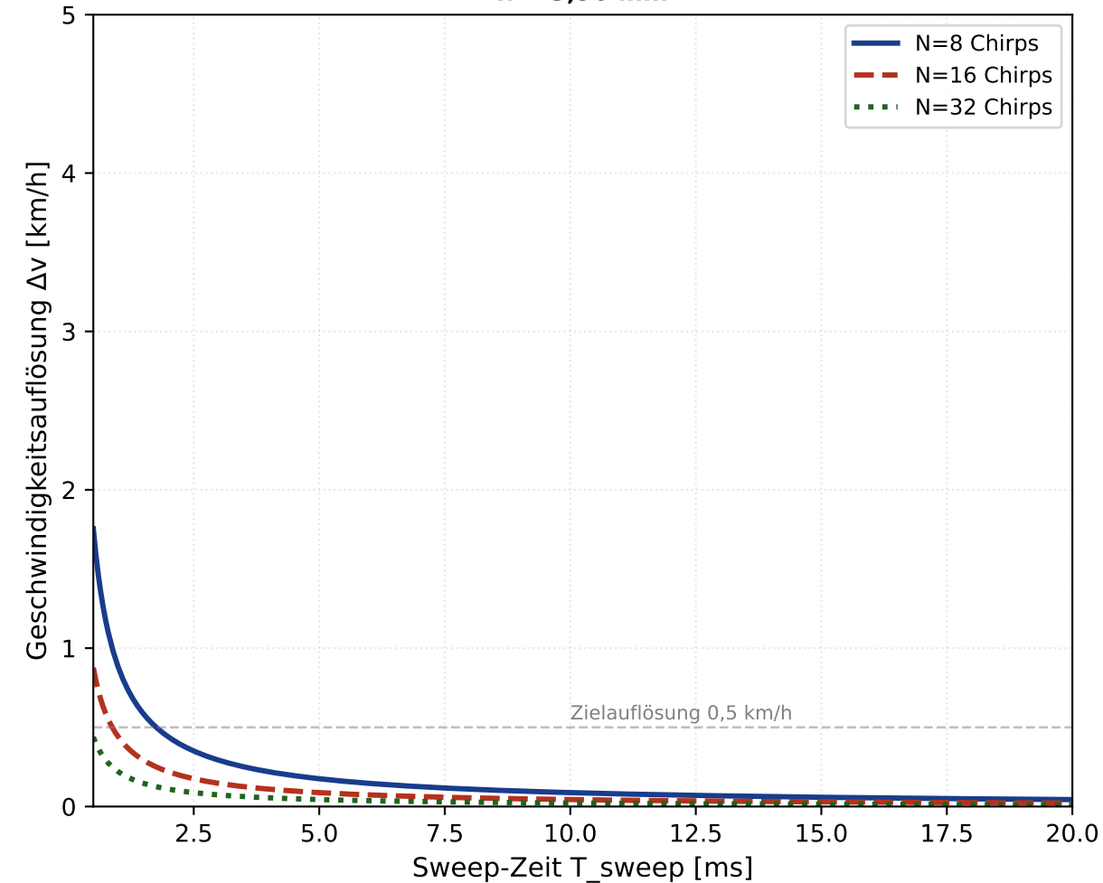
(b) Geschwindigkeitsauflösung 77 GHz FMCW \lambda = 3,90 \text{ mm}
