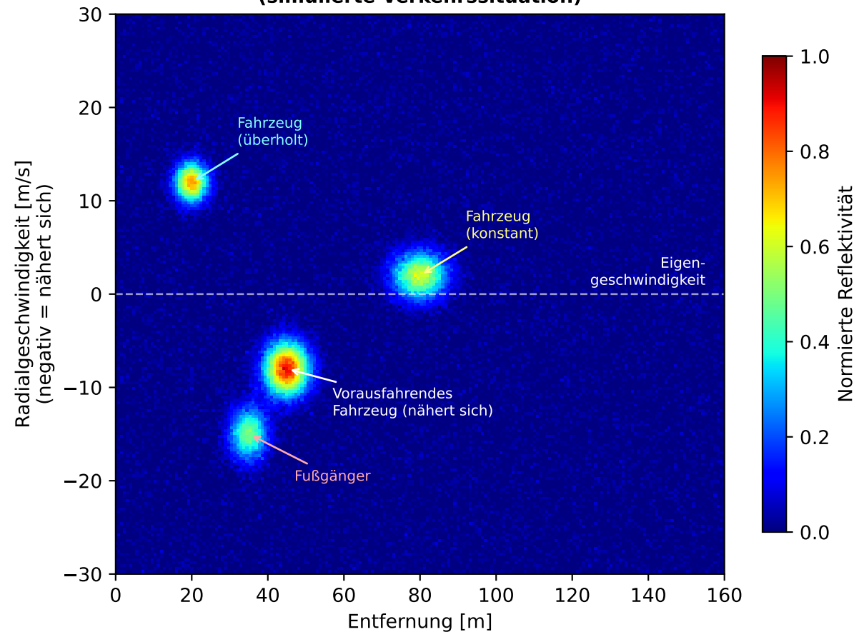
Range-Doppler-Karte: Front-Radar (simulierte Verkehrssituation)
