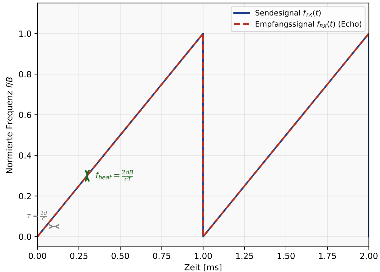
FMCW-Radar: Chirp-Signale und Schwebungsfrequenz (77 GHz, BW = 1 GHz, Ziel bei 30 m)
