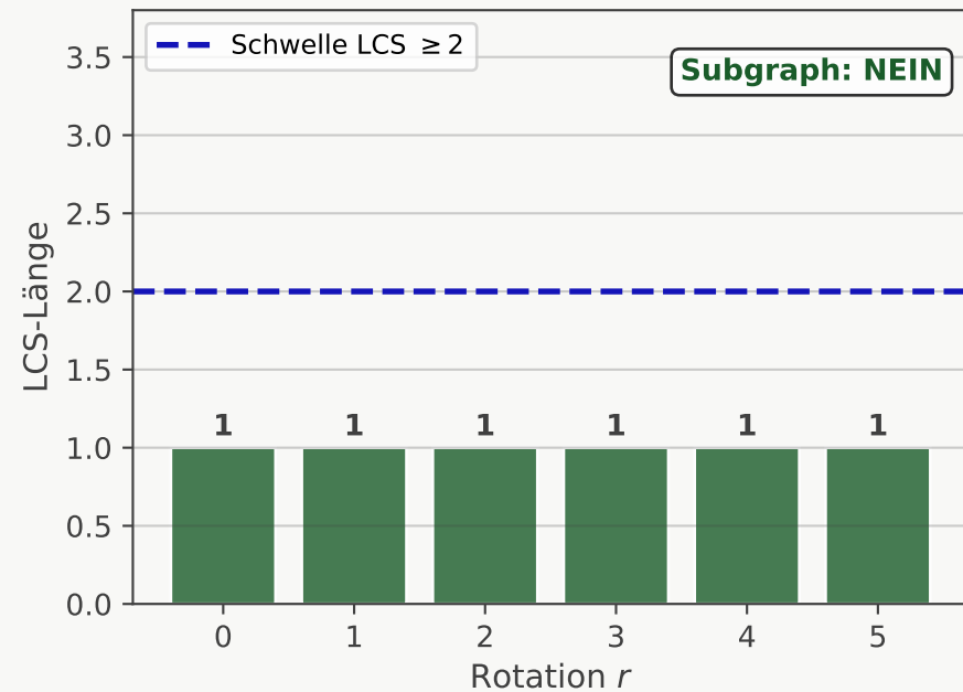
Motiv M_3 \subseteq \mathcal{N}^+ ?
