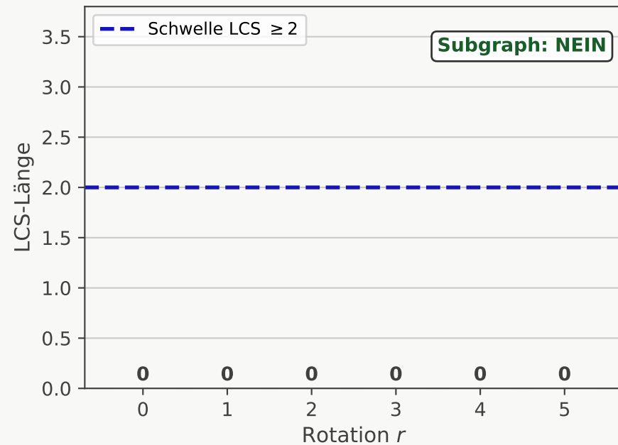
Motiv M_1 \subseteq \mathcal{N}^+ ?
