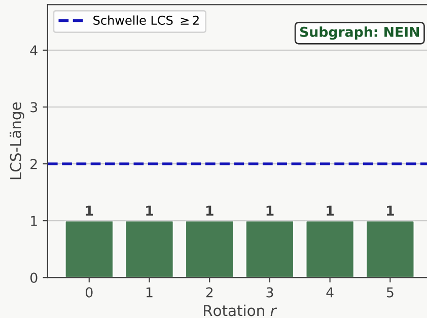
Motiv M_2 \subseteq \mathcal{N}^+ ?
