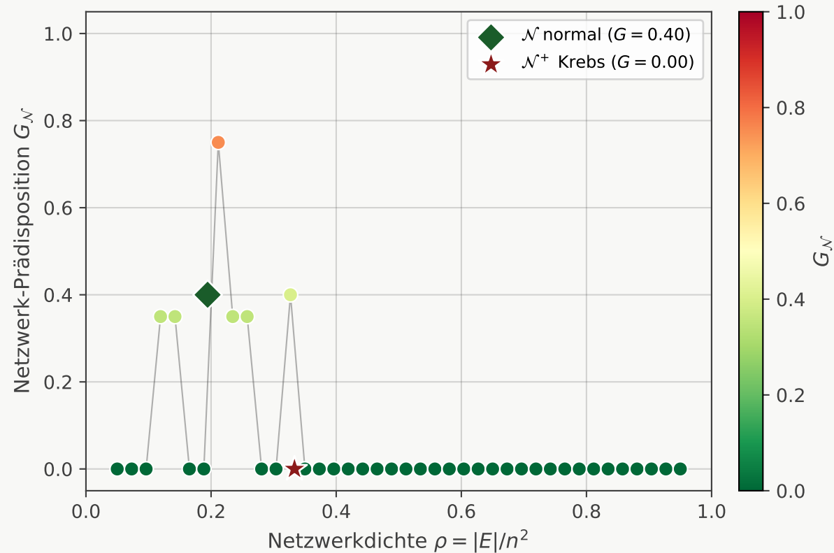
G_{\mathcal{N}} als Funktion der Netzwerkdichte
