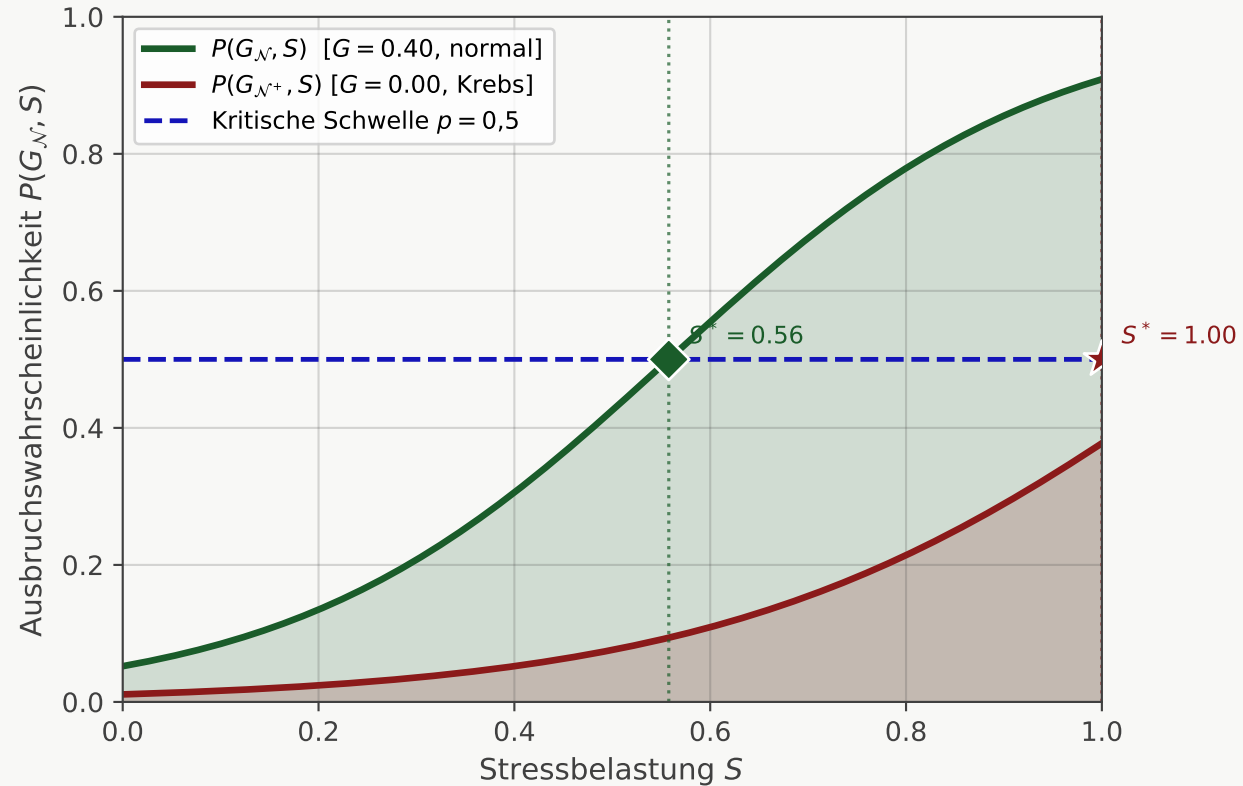
GSKA-Modell mit netzwerk-induziertem G_{\mathcal{N}}
