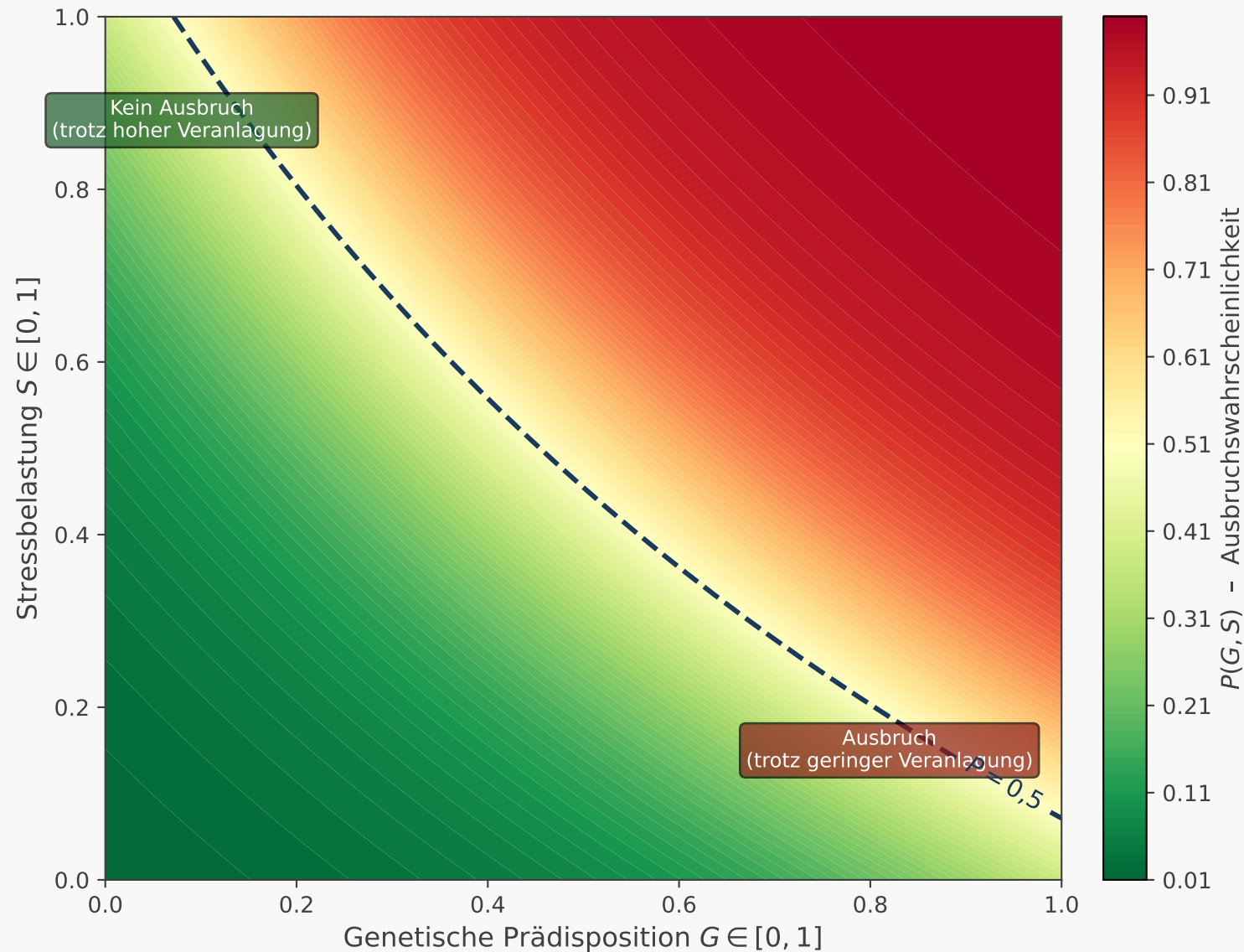
Heatmap der Krebsausbruch-Wahrscheinlichkeit P(G, S)
