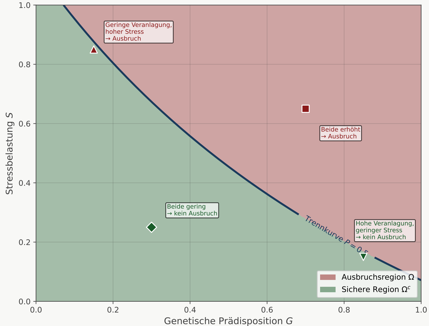
Phasendiagramm: Ausbruchsregion \Omega und komplementäre Region \Omega^c
