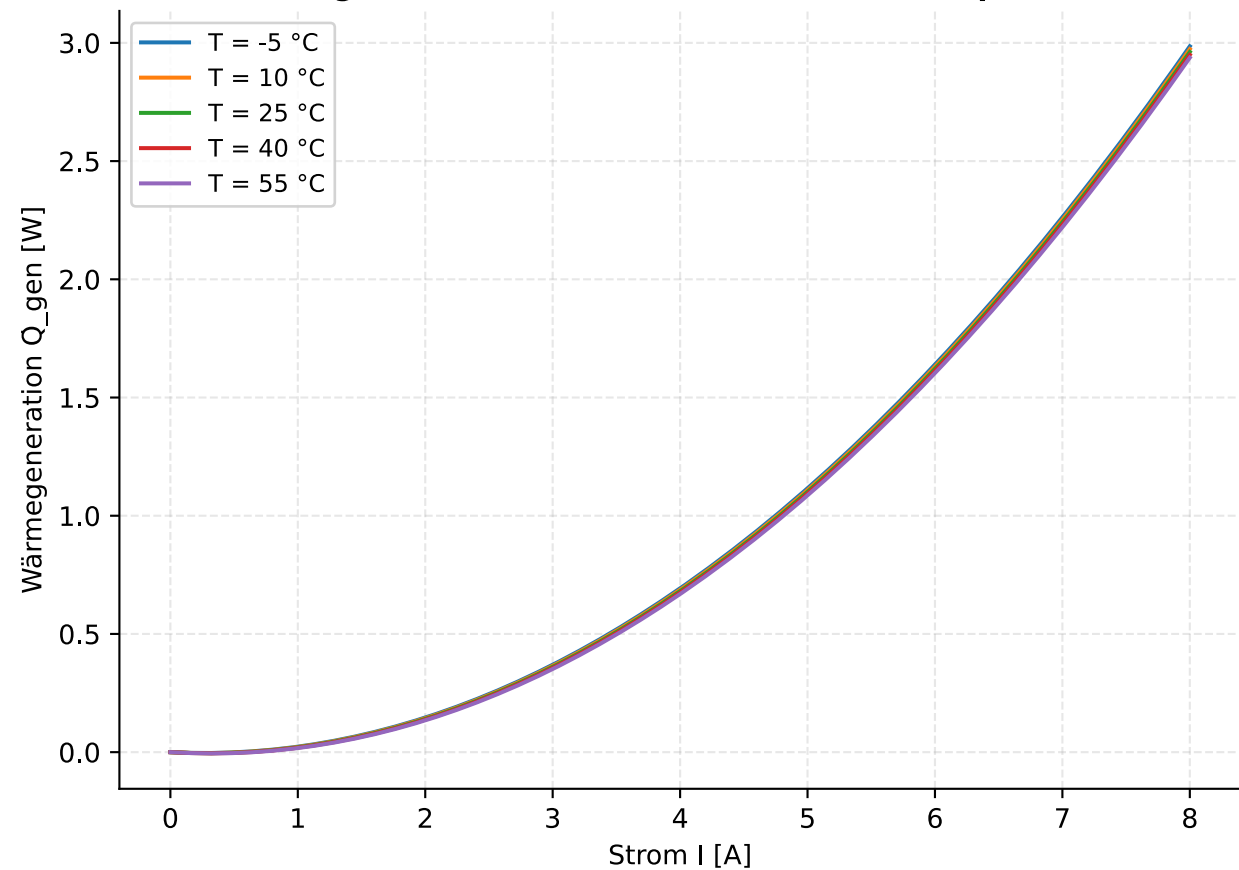
Wärmegeneration Q(I) bei verschiedenen Temperaturen
