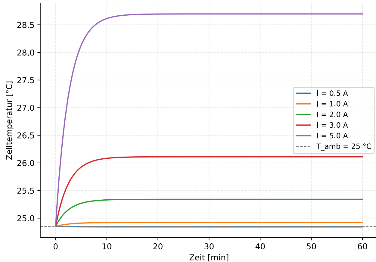
Temperaturverlauf bei konstantem Strom (1 h)
