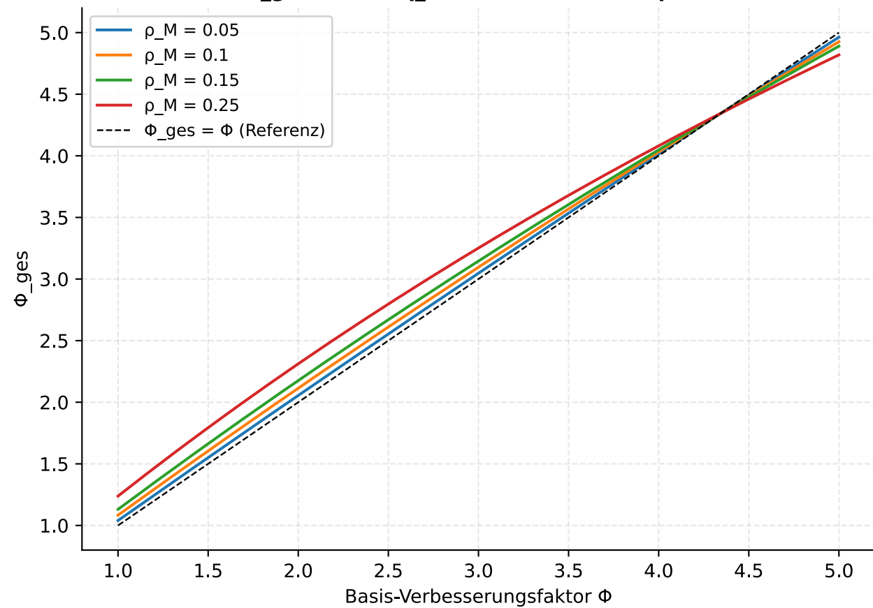
\Phi_{\text{ges}} vs. \Phi ( \eta_{\text{M}} = 0.230 , NMC/Graphit)
