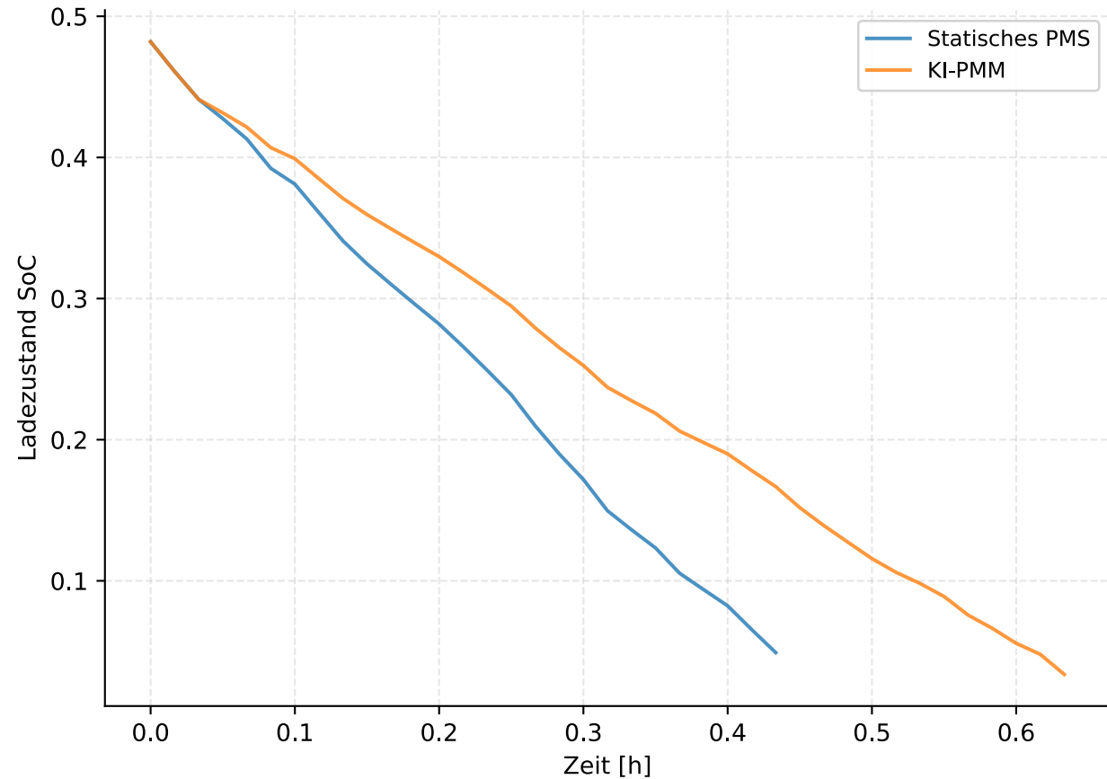
SoC-Verlauf LP2 (E-Bike)
