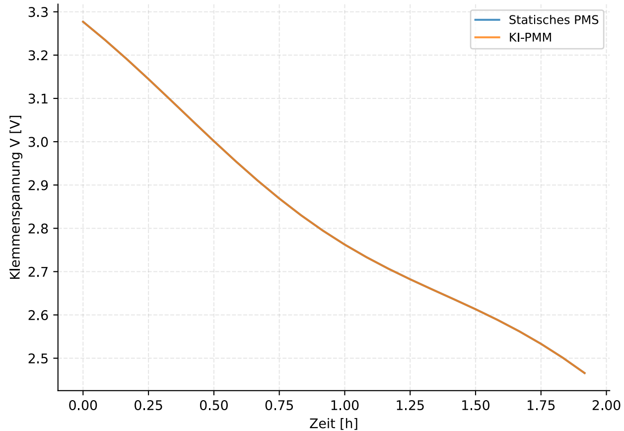
Spannungsverlauf LP3 (Stationär)
