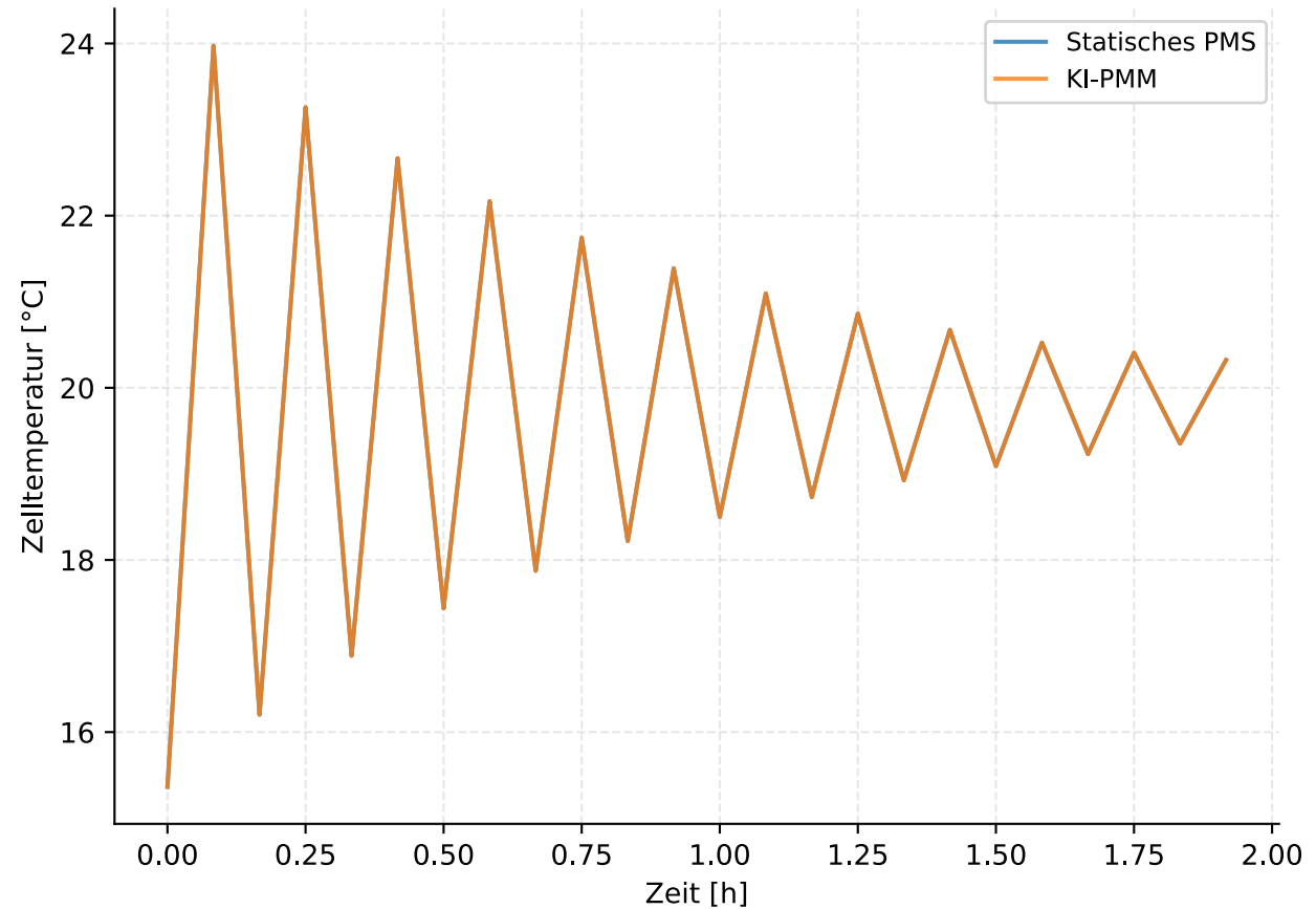
Temperaturverlauf LP3 | T_stat = 19.8 °C | T_AI = 19.8 °C
