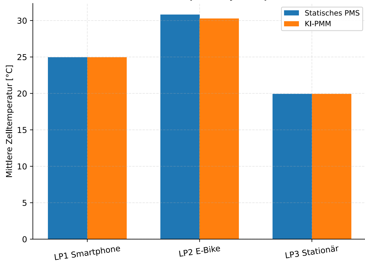
Mittlere Zelltemperatur je Lastprofil
