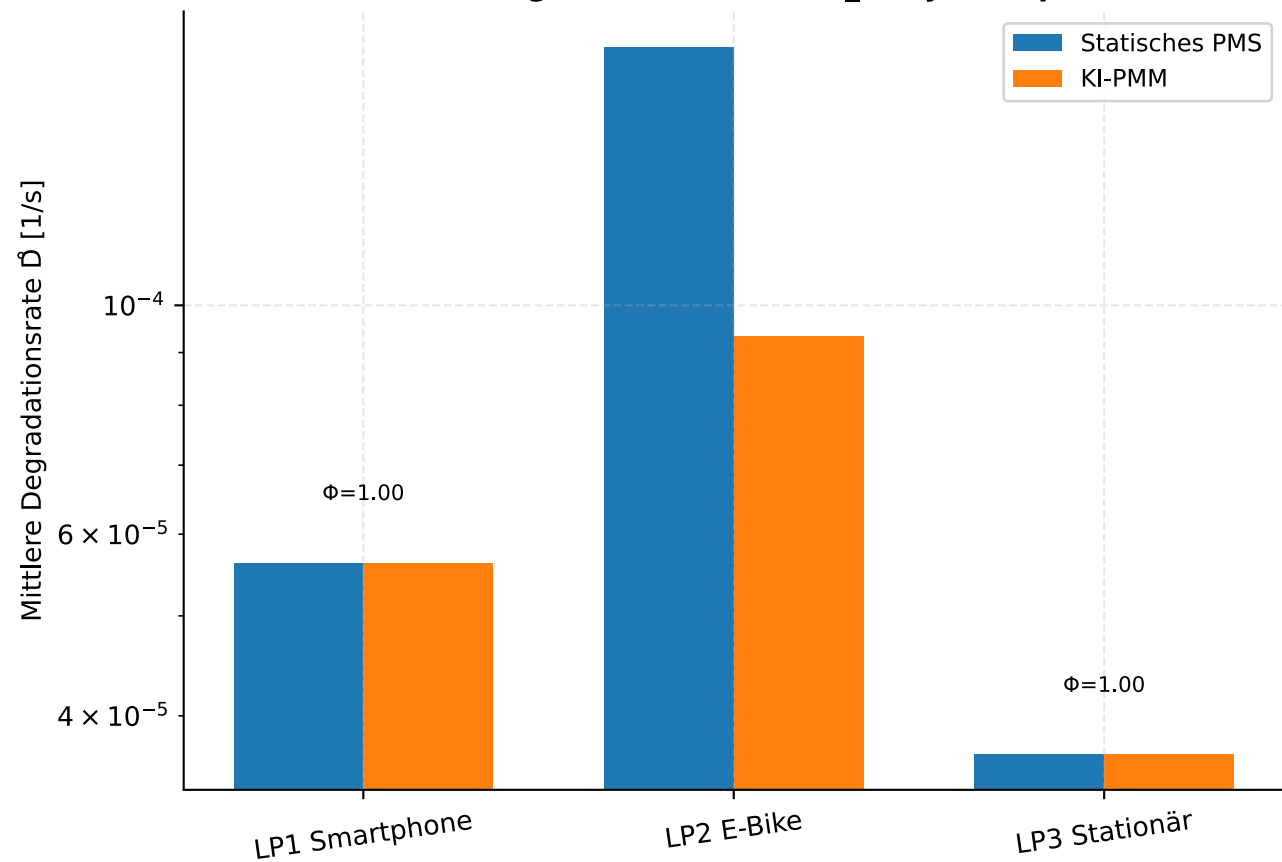
Mittlere Degradationsrate & \Phi_{sim} je Lastprofil
