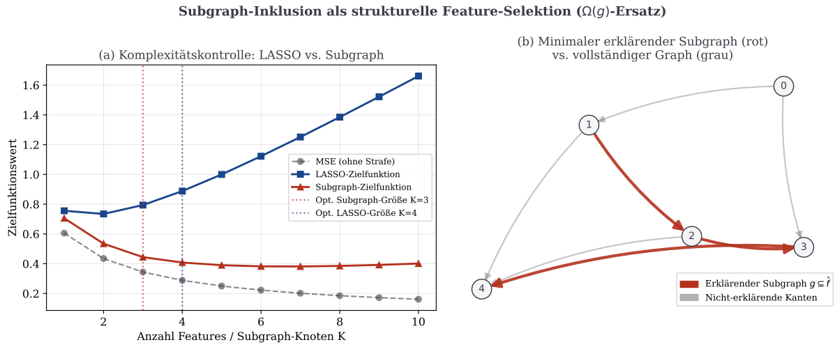
Abbildung 4: (a) Zielfunktionswerte als Funktion der Modellgröße K : Die Subgraph-Zielfunktion (rot) wählt ein kleineres, strukturell konsistenteres Modell ( K = 3 ) als LASSO ( K = 4 ), da sie Kanten außerhalb des Subgraphs stark bestraft. (b) Minimaler erklärender Subgraph (rote Kanten) für eine Vorhersage: Nur die für die Entscheidung relevanten Kanten werden behalten, während nicht-erklärende Verbindungen (grau) ausgeblendet werden.
