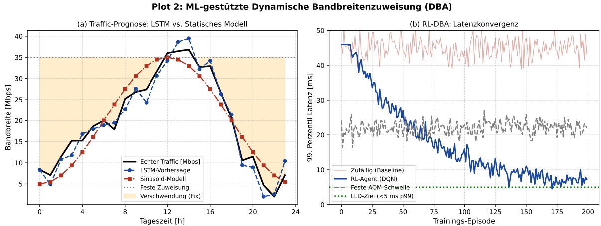
Figure 2: ML-gestützte DBA. (a) Tages-Traffic-Prognose: LSTM-Modell (blau, gestrichelt) approximiert den echten Traffic (schwarz) wesentlich genauer als das sinusoidale Basismodell (rot), insbesondere bei unerwarteten Lastspitzen. Die orange Fläche zeigt die Verschwendung bei fixer Zuweisung (grau gepunktet). (b) RL-DBA-Latenzkonvergenz über Trainings-Episoden: Der DQN-Agent (blau) lernt, die p99-Latenz von initial über 40ms auf unter 5 ms (grüne LLD-Grenze) zu reduzieren, während die feste AQM-Schwelle (grau) dauerhaft über dem Ziel verbleibt.
