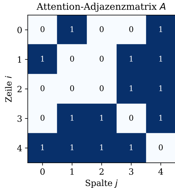
Plot 3: Signaturberechnung für Transformer-Attention-Matrix
