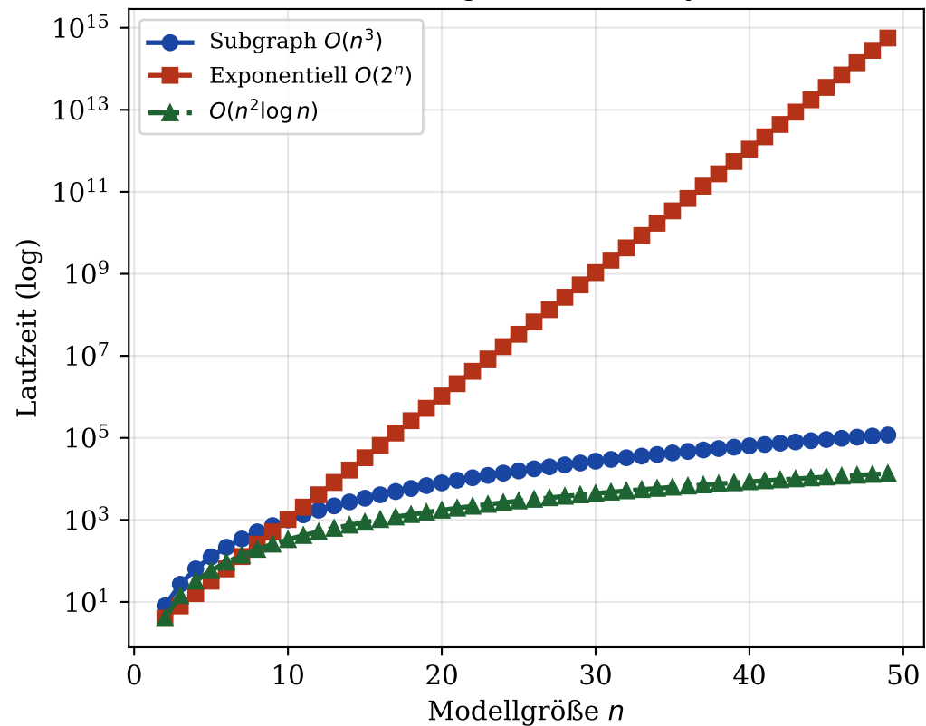
Skalierung für LLM-Analyse
