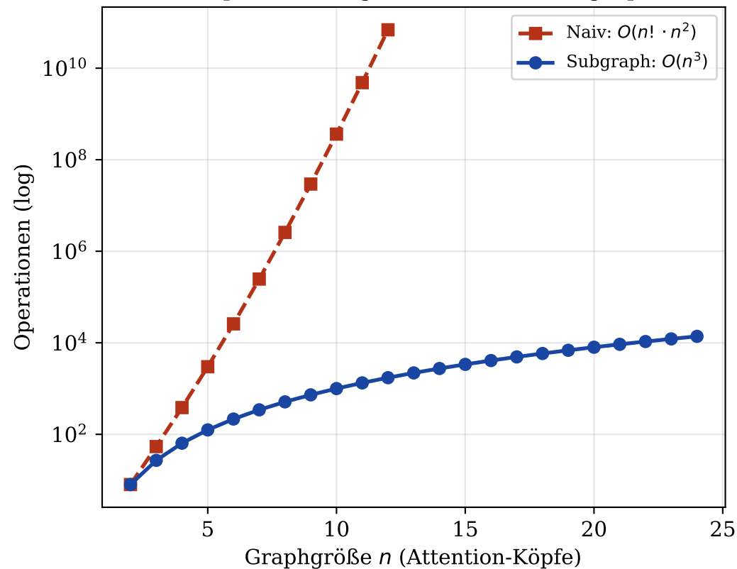
Komplexitätsvergleich: Naiv vs. Subgraph
