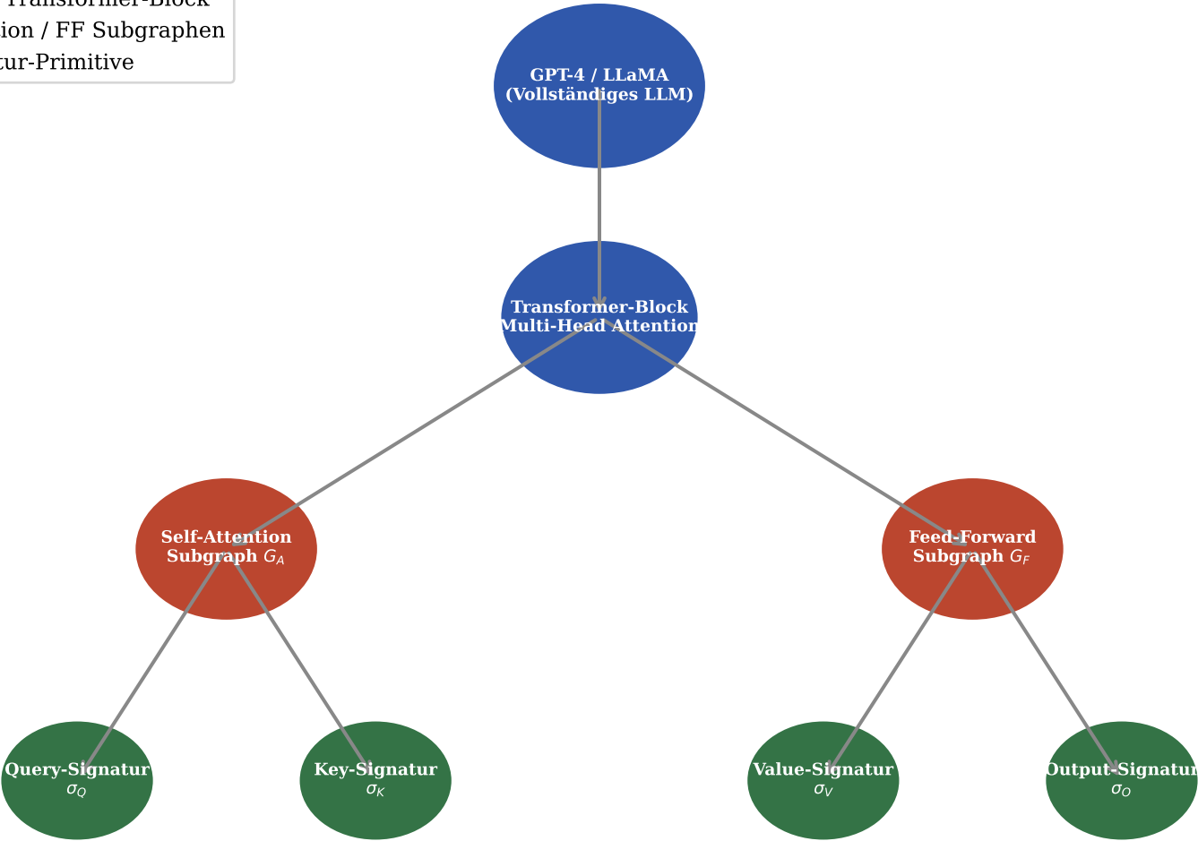
Plot 7: Hierarchische Subgraph-Zerlegung eines LLM
