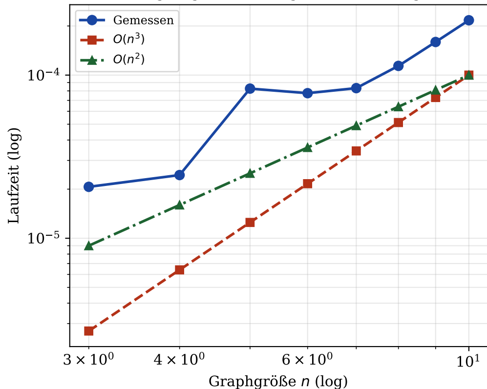
Log-Log-Darstellung der Skalierung
