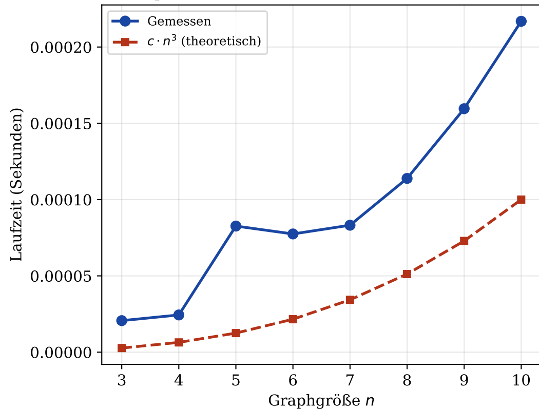
Empirische Laufzeit vs. theoretische Schranke
