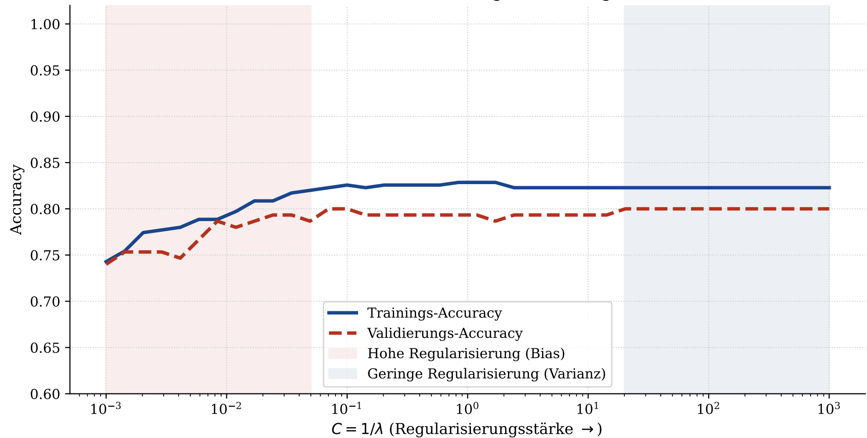
Bias-Varianz-Tradeoff bei logistischer Regression
