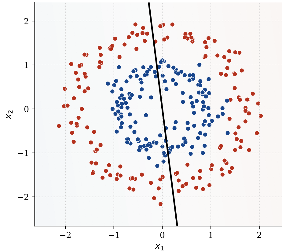
Kreisförmige Daten Accuracy: 49.67%
