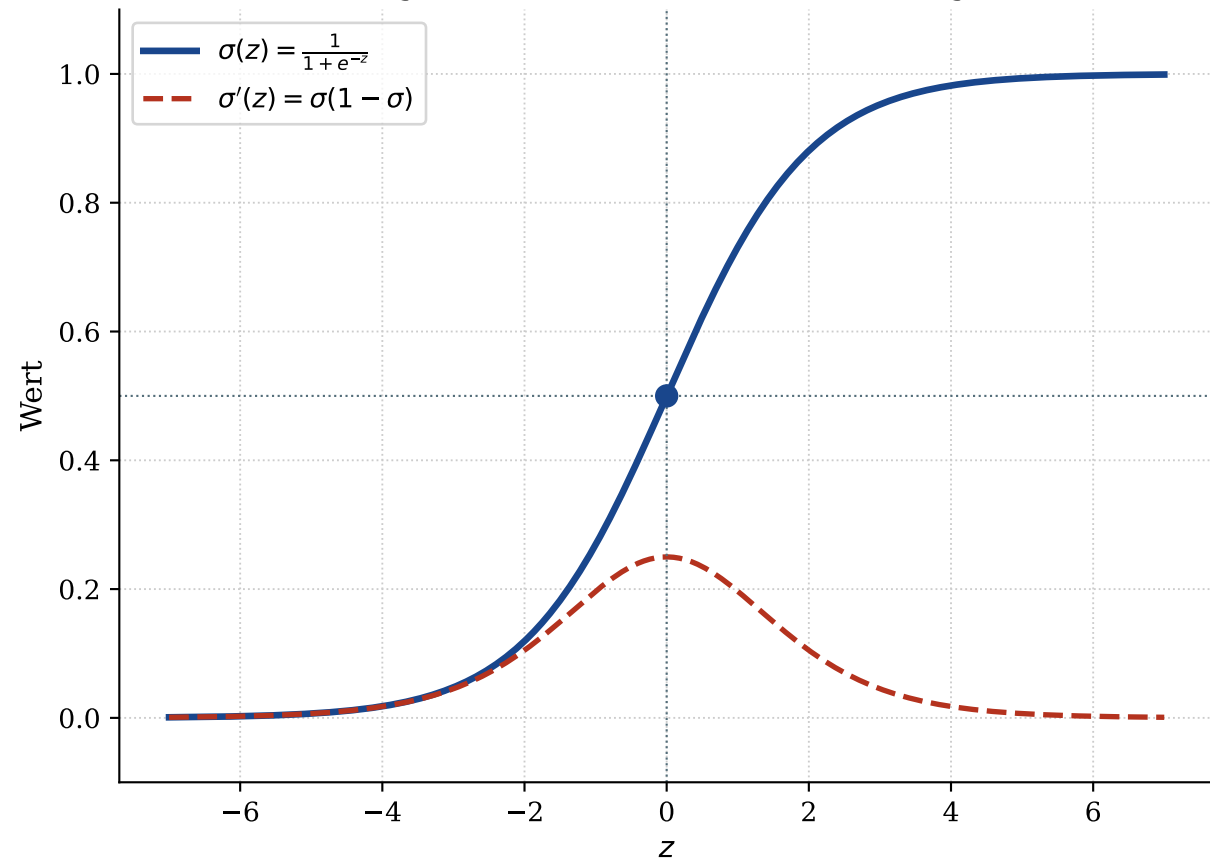
Sigmoid-Funktion und ihre Ableitung
