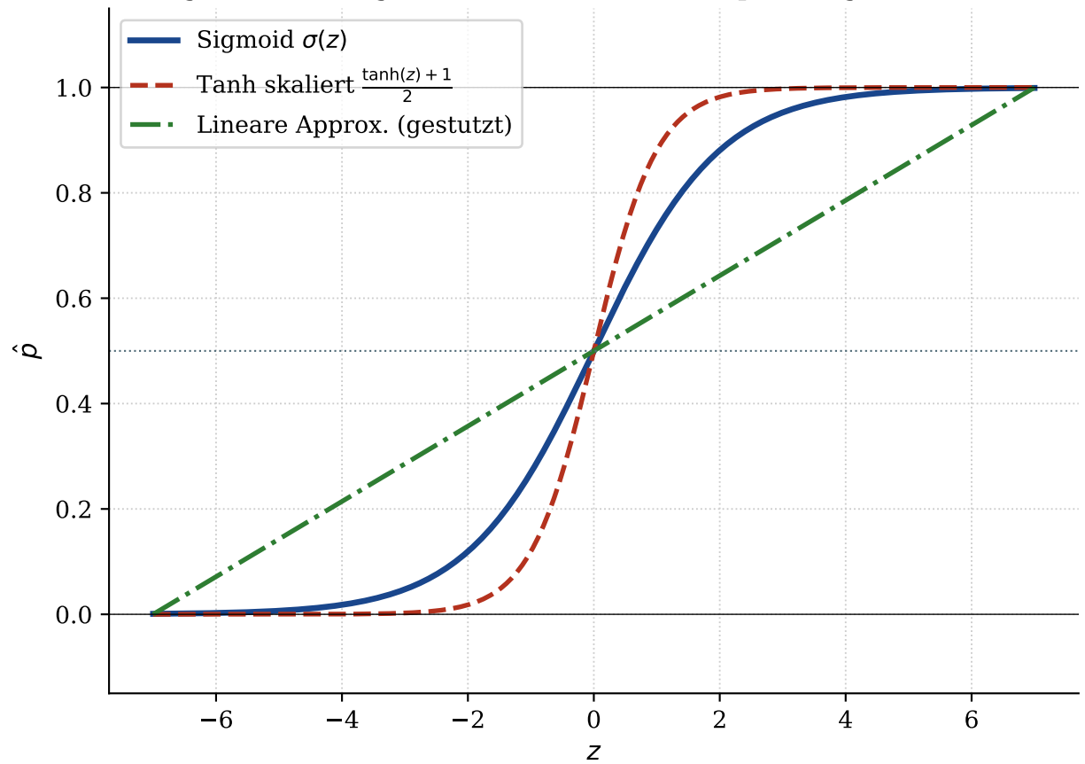
Sigmoid im Vergleich mit alternativen Squashing-Funktionen
