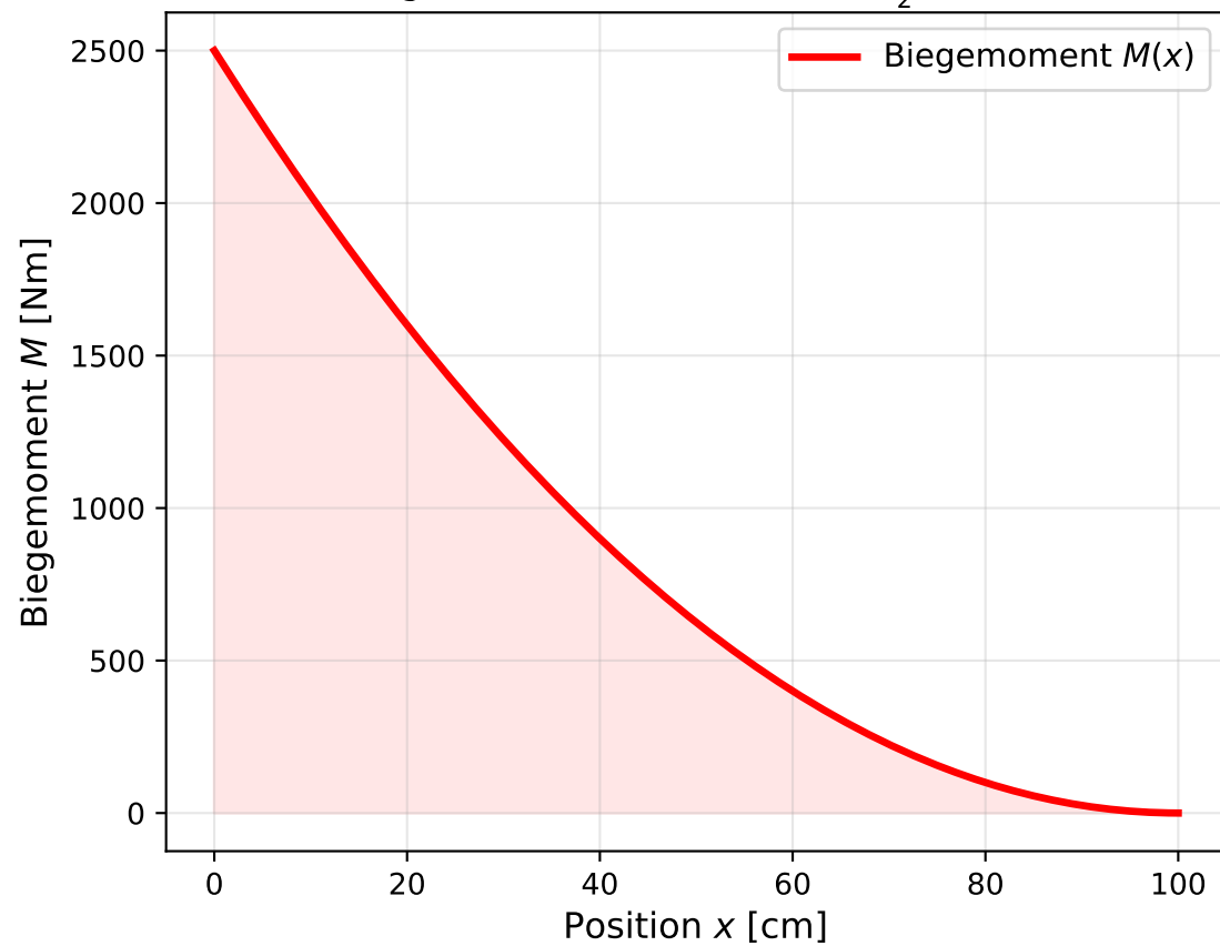
Biegemomentenverlauf M(x) = \frac{q}{2}(L - x)^2
