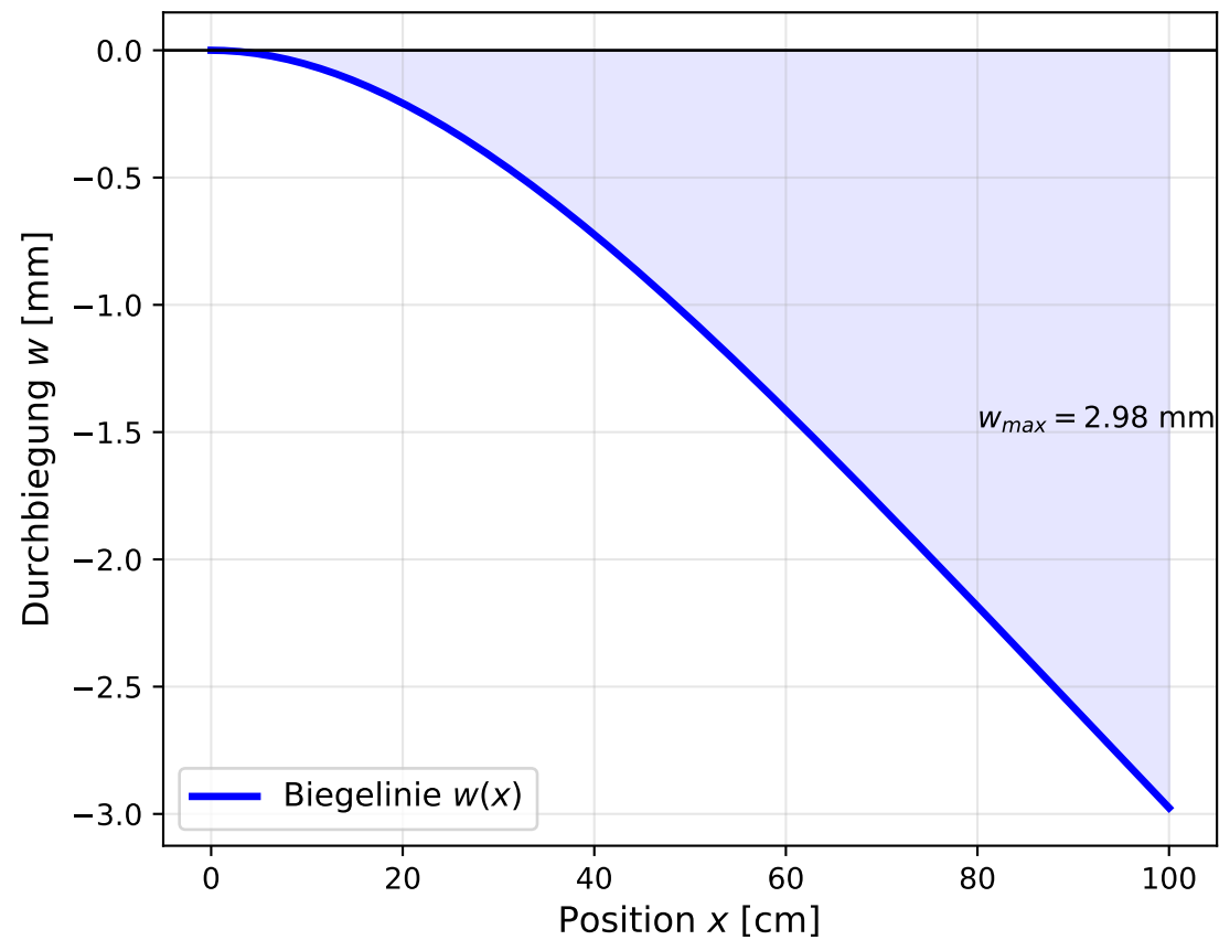
Kragarm mit Gleichstreckenlast q
