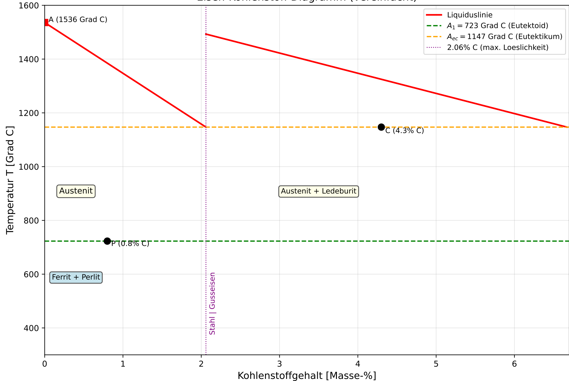
Eisen-Kohlenstoff-Diagramm (vereinfacht)
