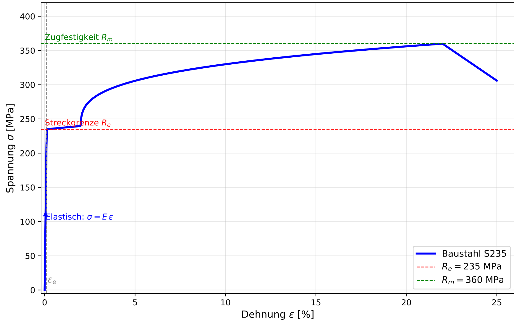
Spannungs-Dehnungs-Diagramm (Zugversuch, Stahl S235)
