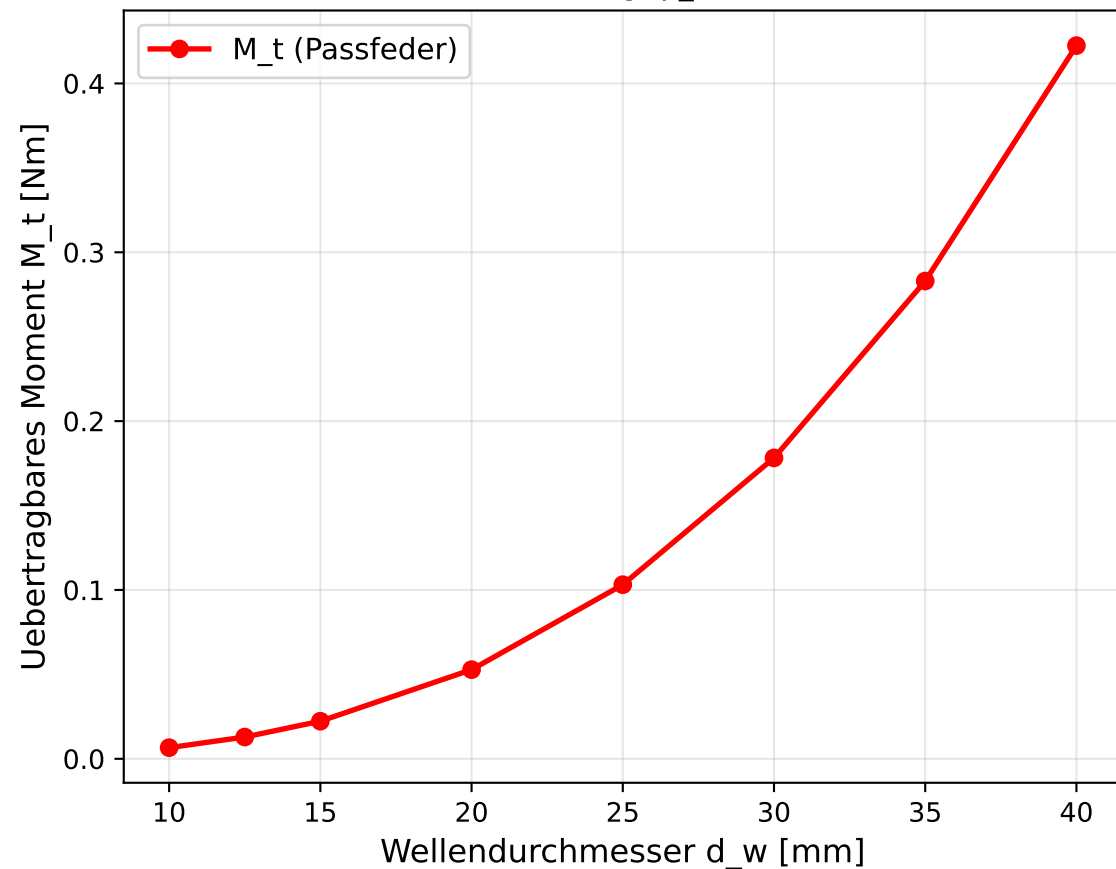
Passfederverbindung ( p_{zul} = 100 MPa)
