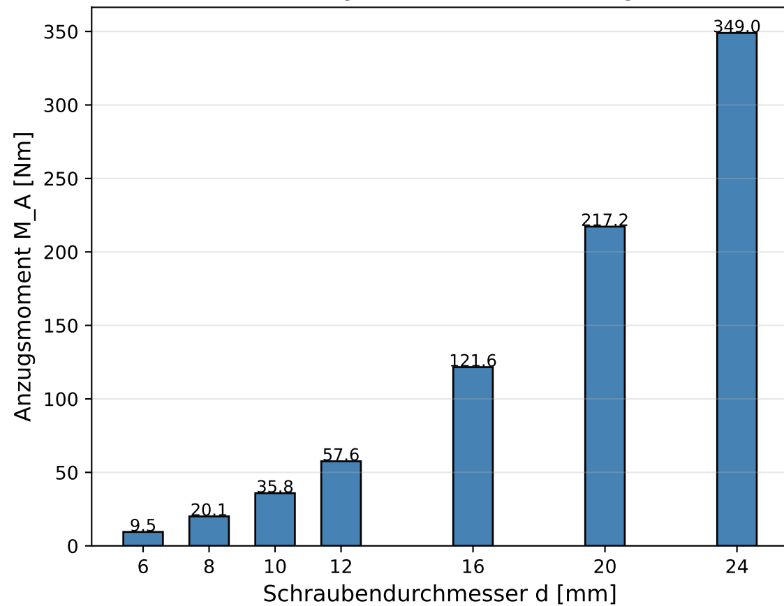
Richtwerte Anzugsmoment ( \mu=0.12 , Festigkl. 8.8)
