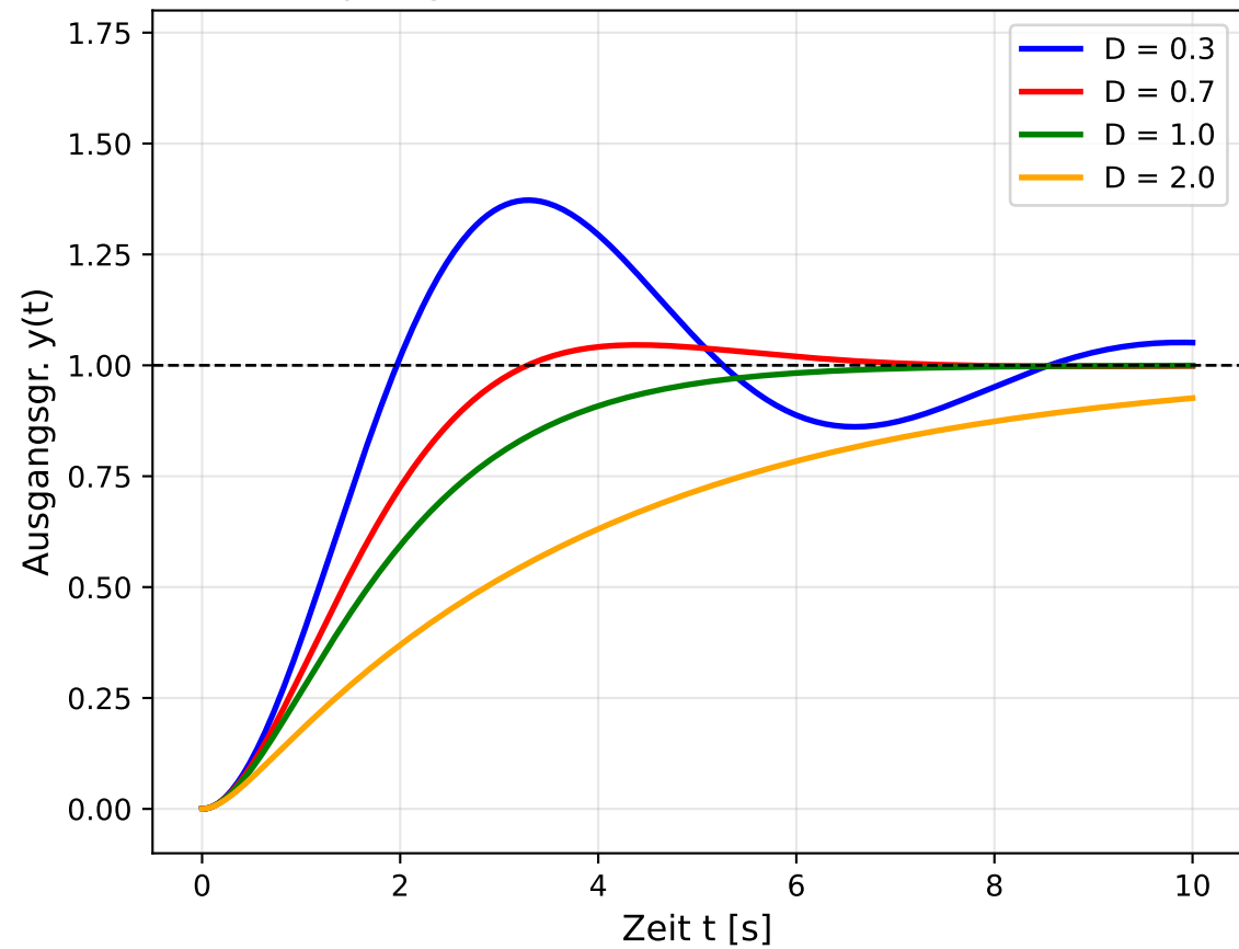
Sprungantwort PT2-Glied (verschiedene D)
