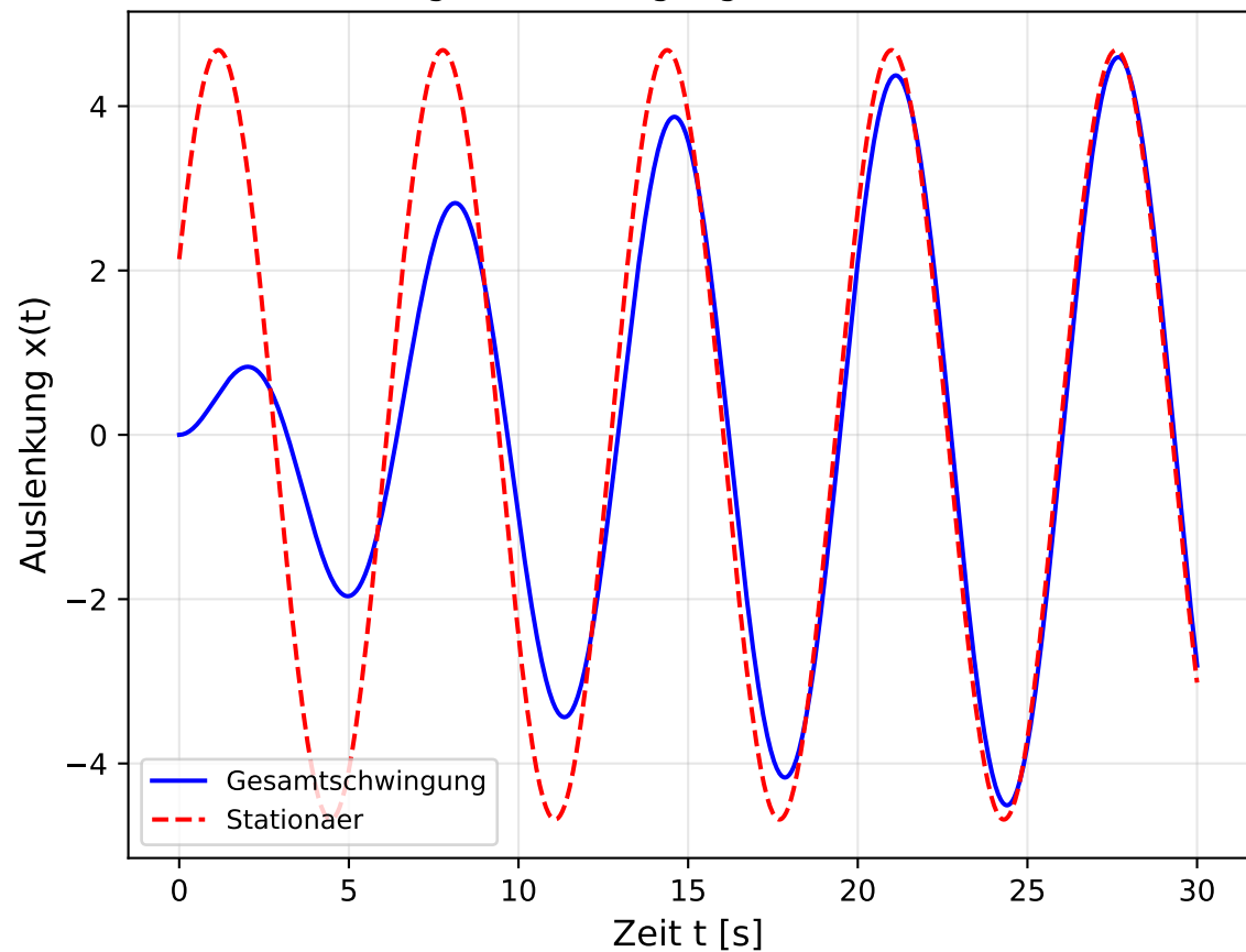
Erzwungene Schwingung ( D=0.1 , \eta=0.95 )
