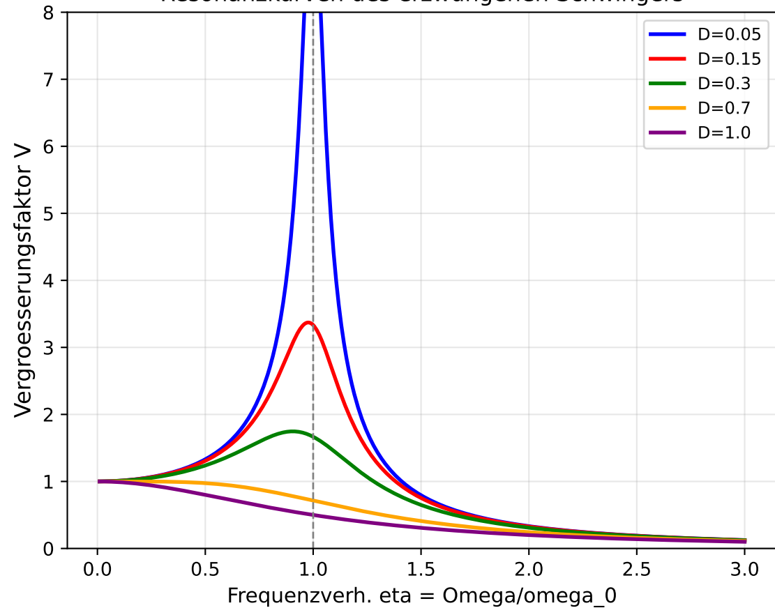
Resonanzkurven des erzwungenen Schwingers
