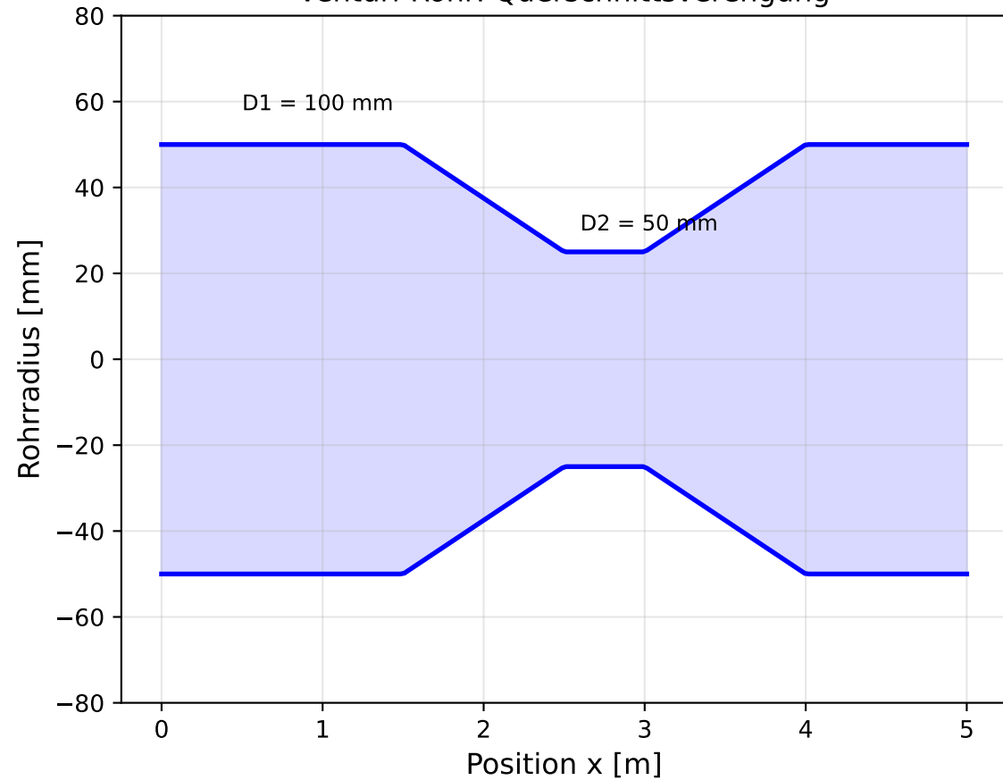
Venturi-Rohr: Querschnittsverengung
