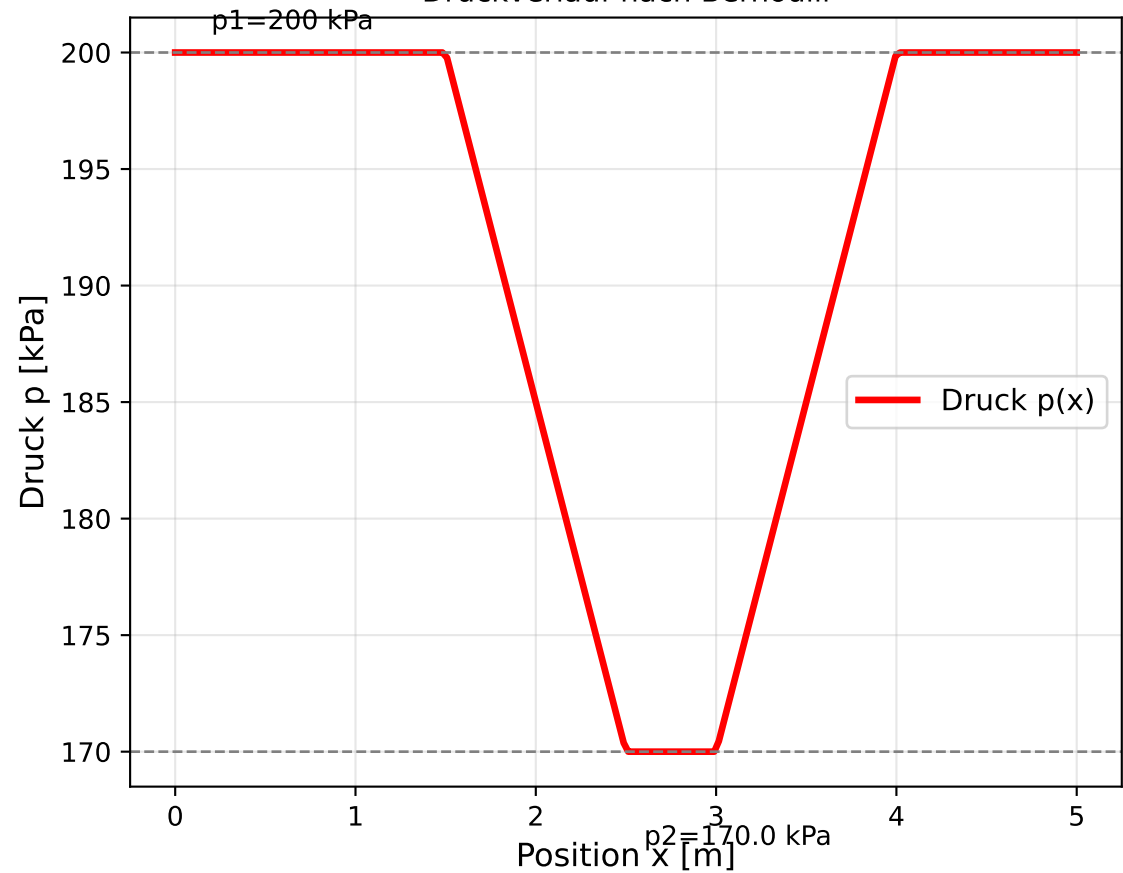
Druckverlauf nach Bernoulli
