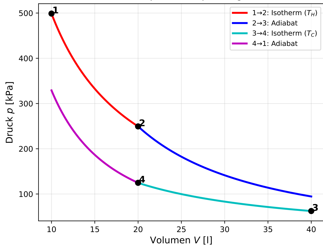
Carnot-Kreisprozess im p - V -Diagramm
