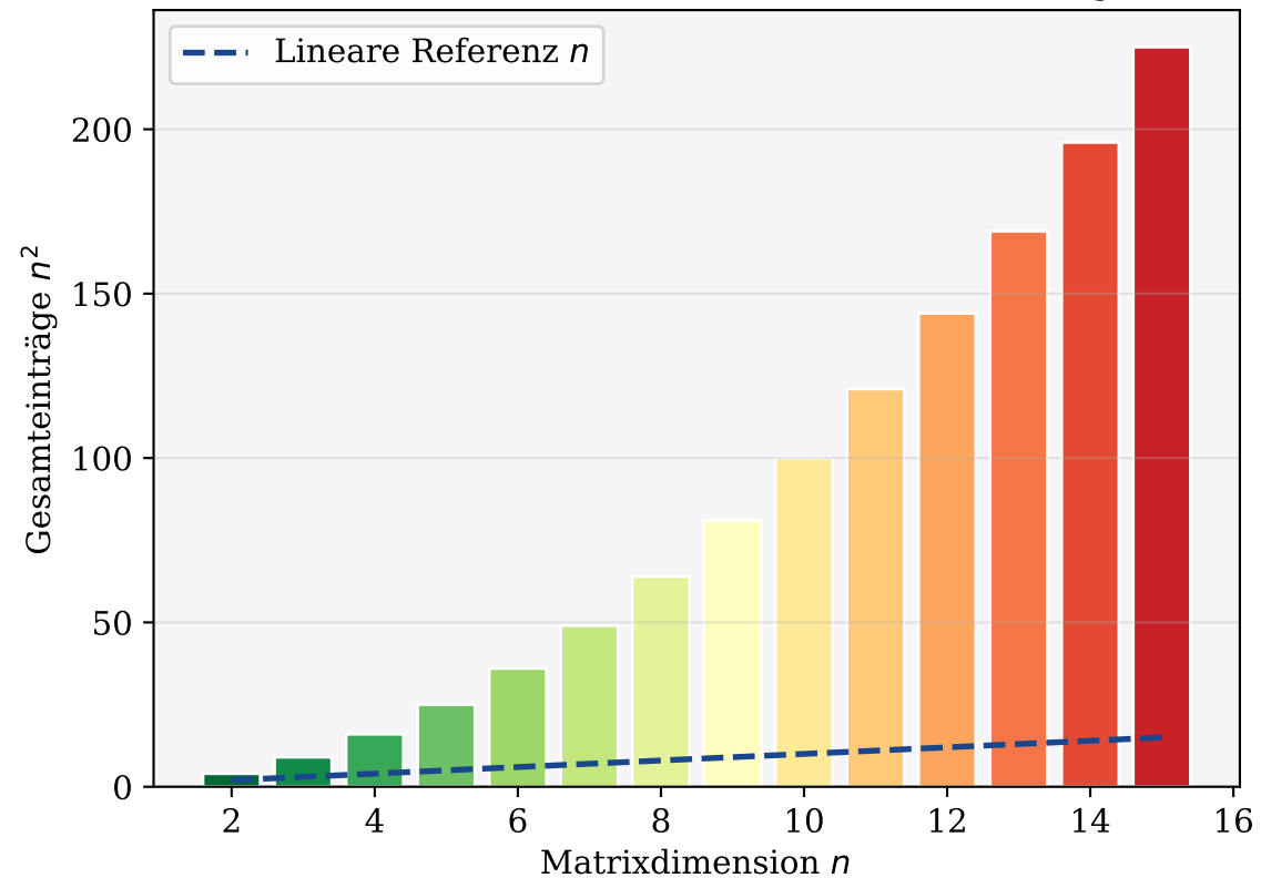
Quadratisches Wachstum der Matrixeinträge
