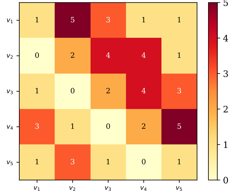
A^4 : Wege der Länge 4
