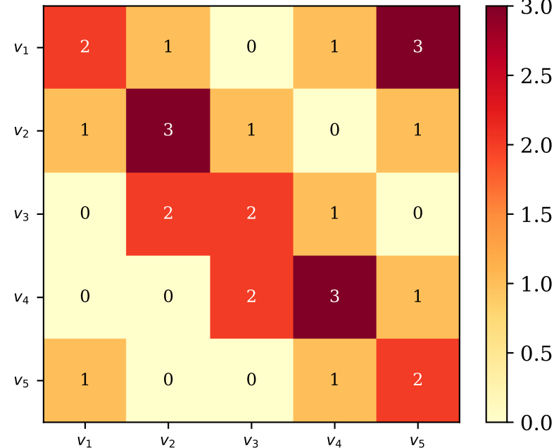
A^3 : Wege der Länge 3
