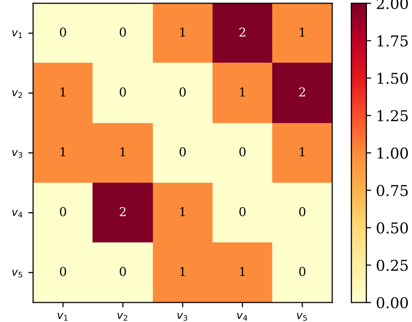
A^2 : Wege der Länge 2
