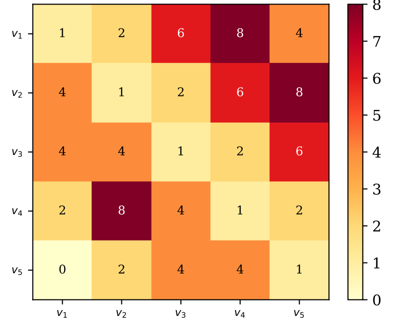
A^5 : Wege der Länge 5
