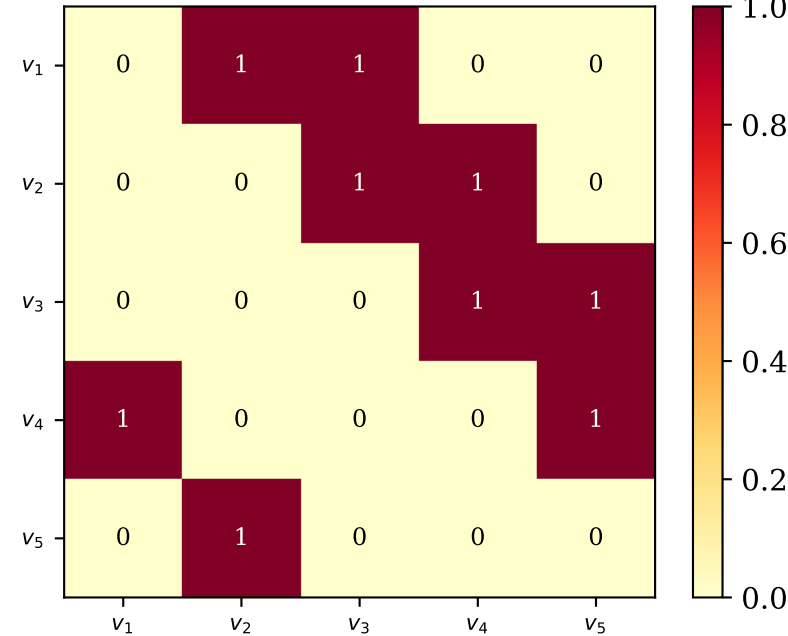
A^1 : Wege der Länge 1
