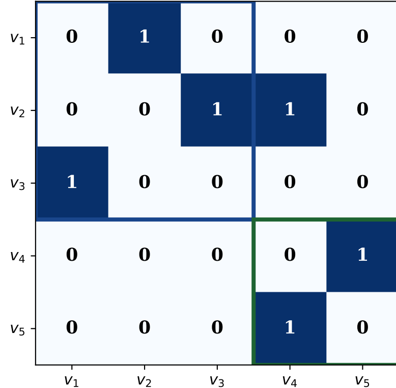
Adjazenzmatrix mit 2 SCCs
