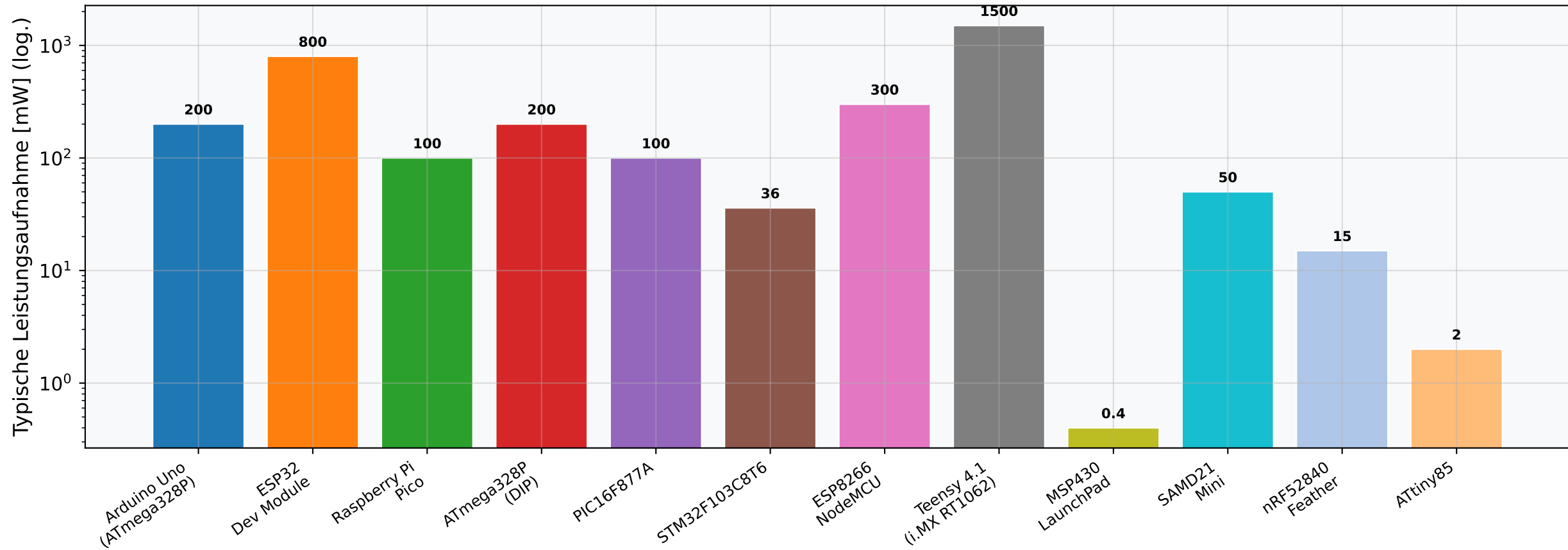
Abbildung 3 – Leistungsaufnahme im Aktivbetrieb
