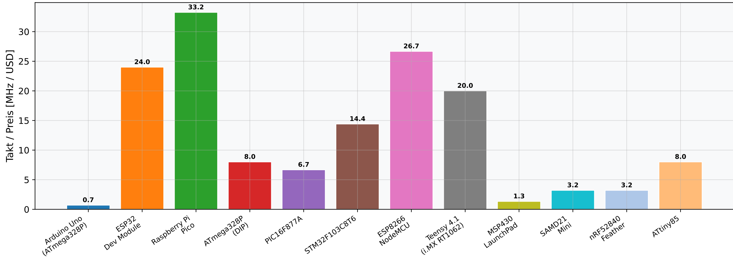
Abbildung 4 – Preis-Leistungs-Verhältnis (Taktfrequenz pro USD)
