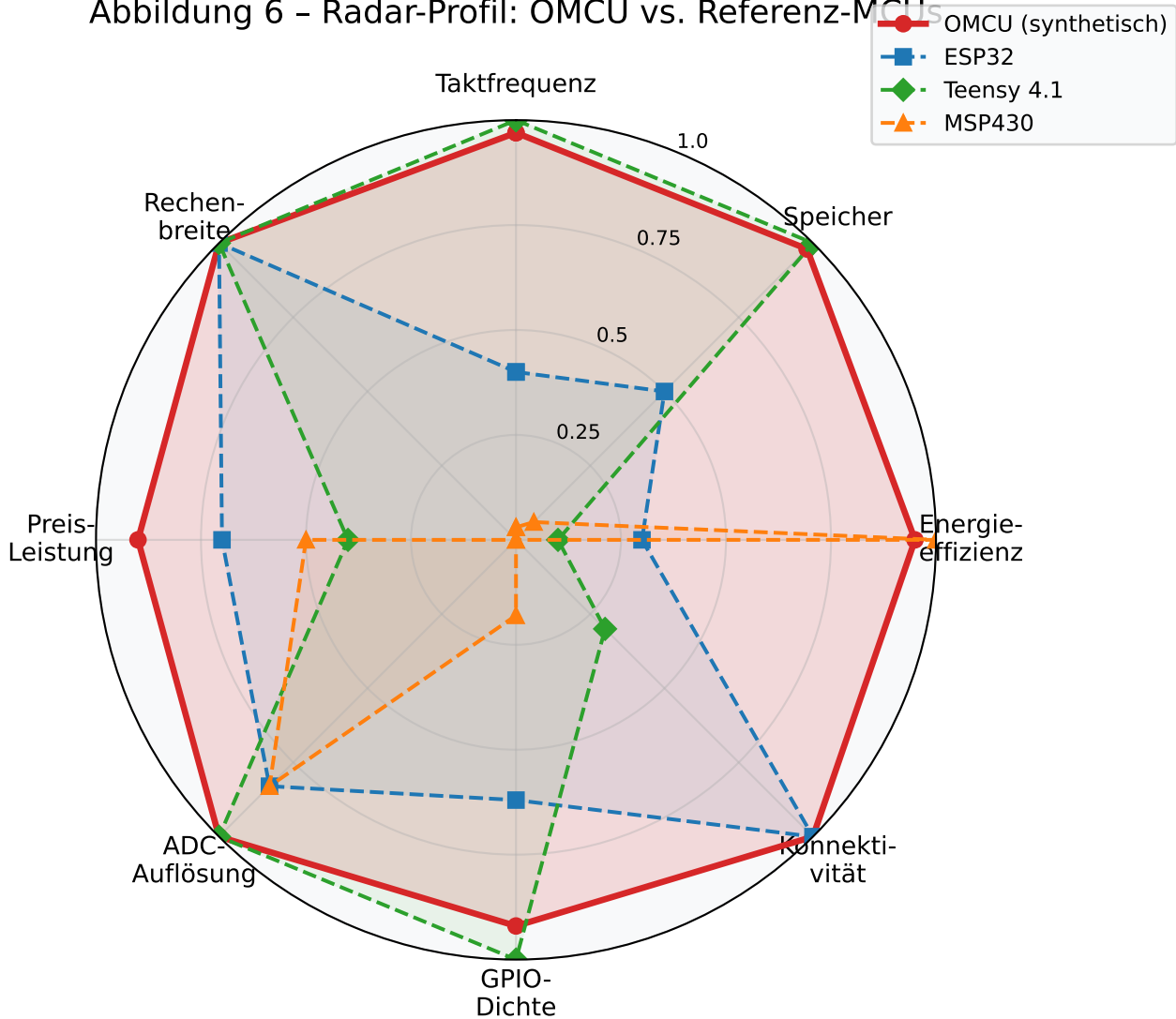
Abbildung 6 - Radar-Profil: OMCU vs. Referenz-MCUs
