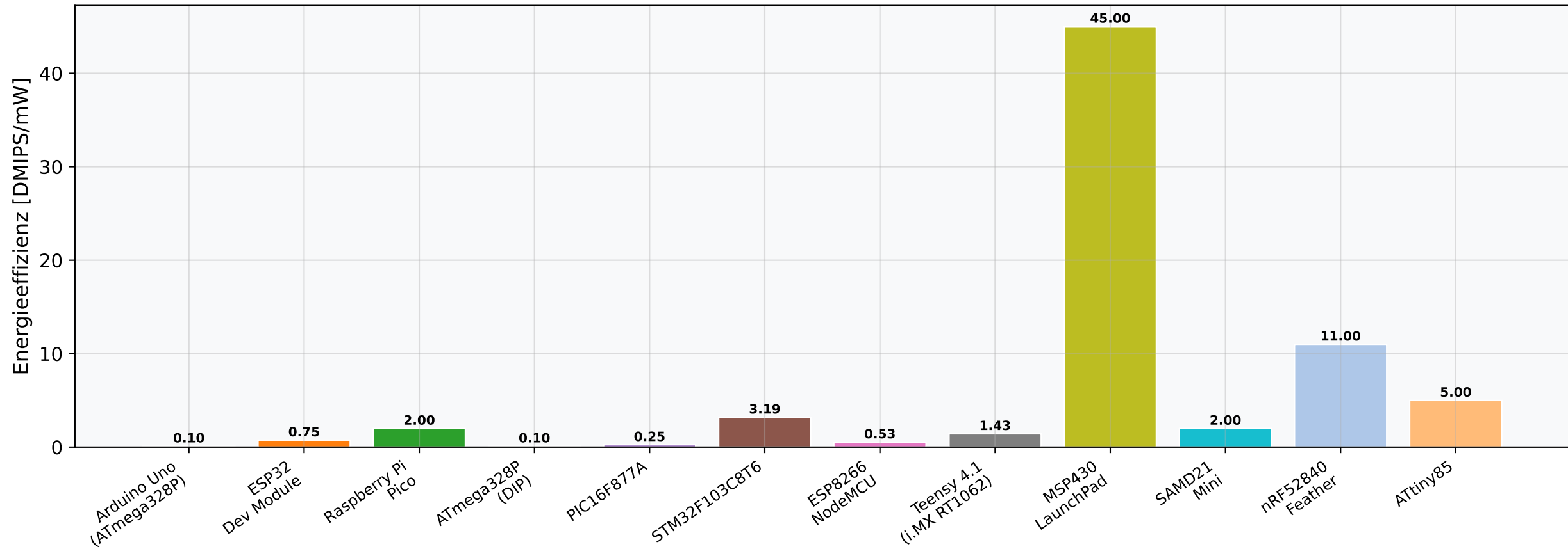
Abbildung 8 – Energieeffizienz: DMIPS pro Milliwatt
