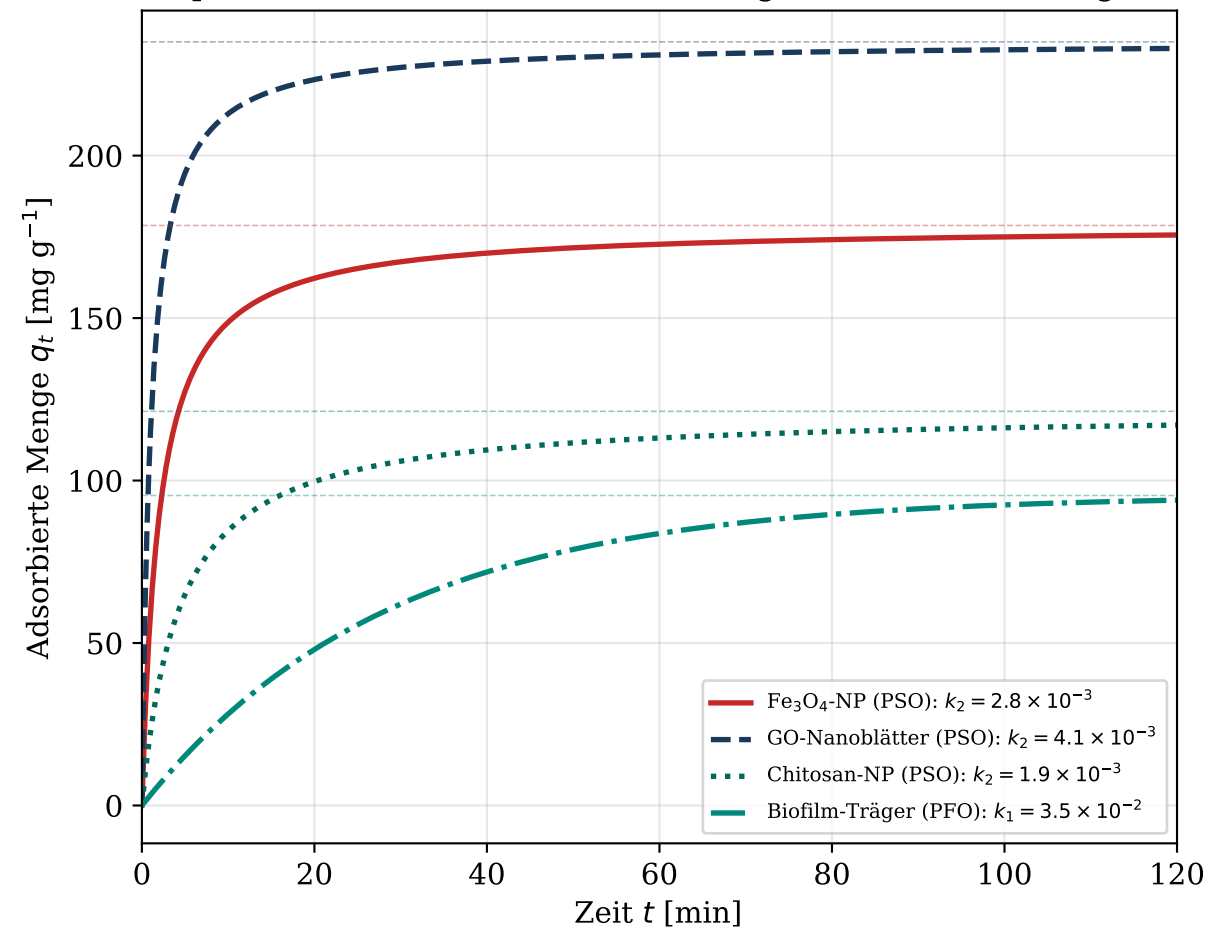
Adsorptionskinetiken: Pseudo-2.-Ordnung (PSO) & 1.-Ordnung (PFO)
