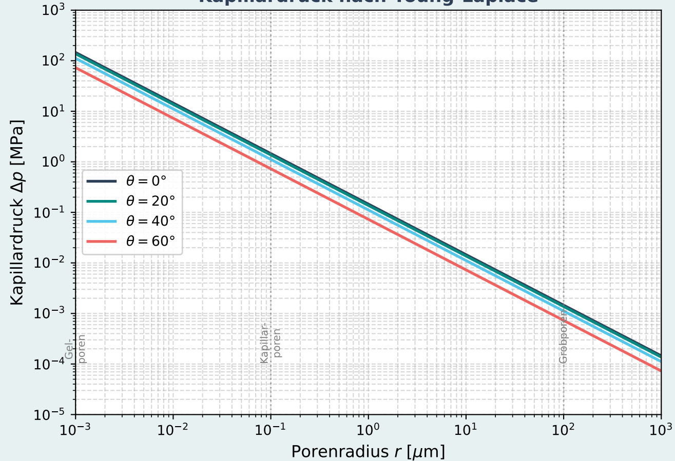
Kapillardruck nach Young-Laplace
