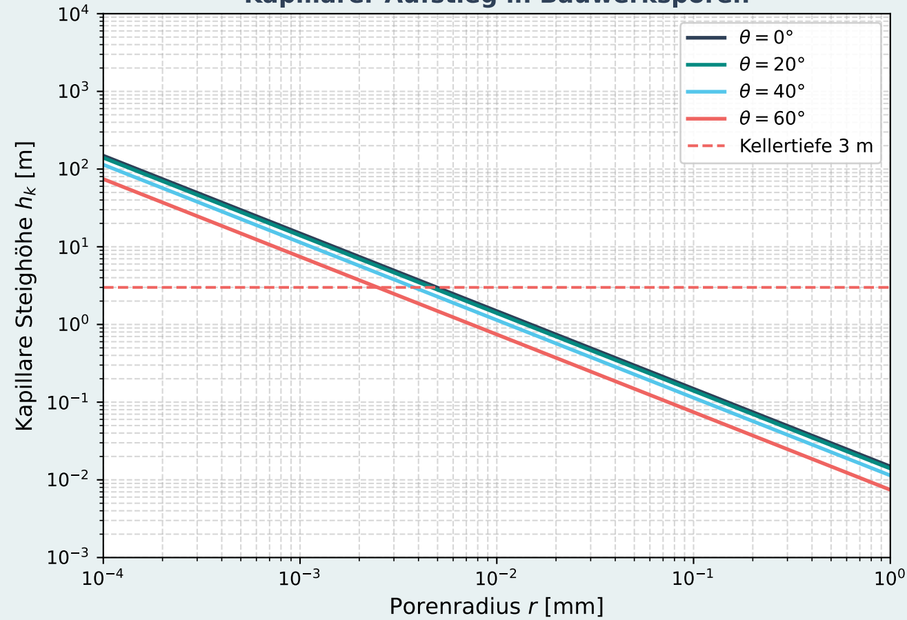
Kapillarer Aufstieg in Bauwerksporen
