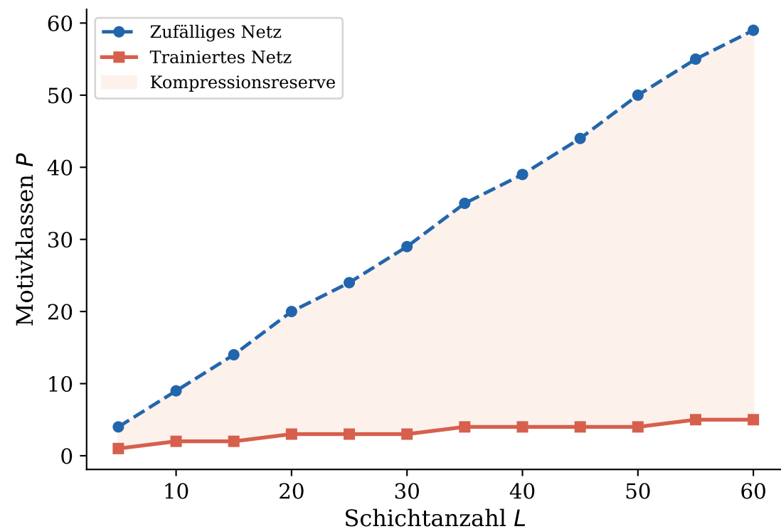
Redundanz in trainierten Netzen
