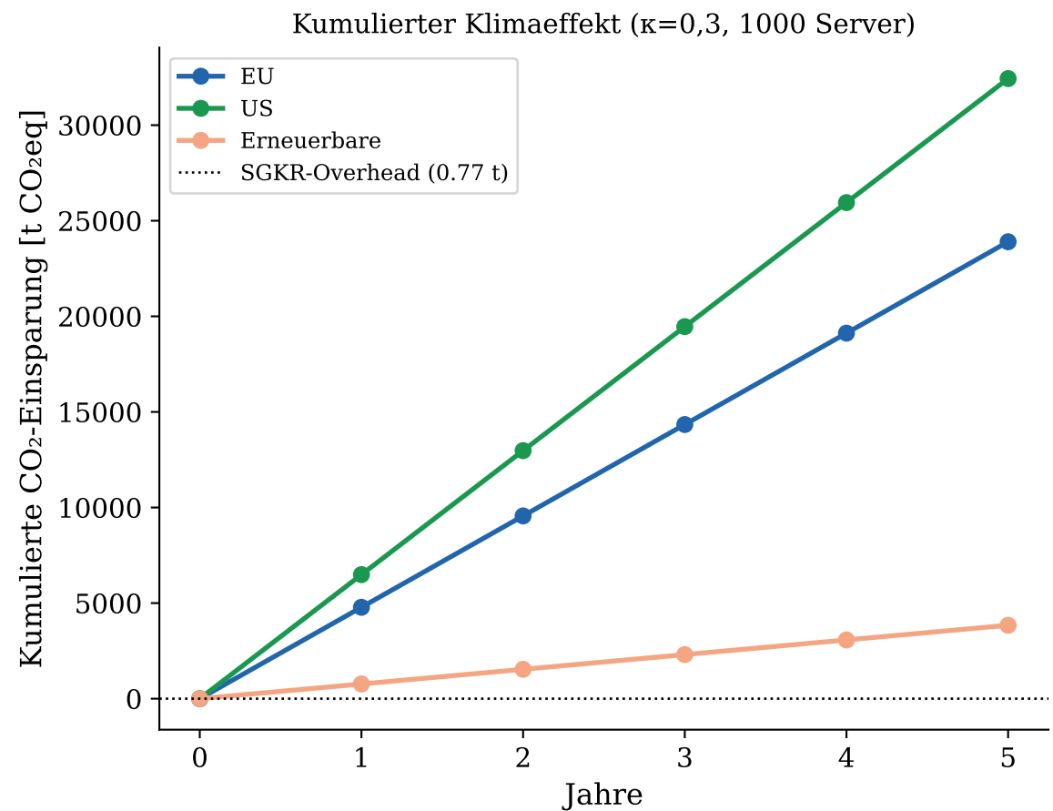
Abb. 18: CO 2 -Bilanz und Klimaimpact durch minimierte neuronale Netze
