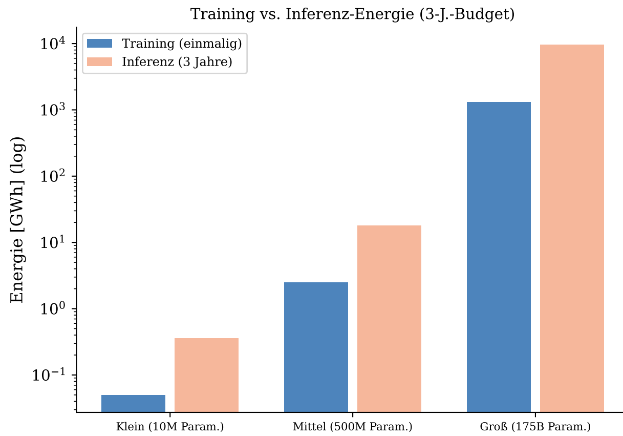
Abb. 21: Modell-Lebenszyklus-Energieanalyse: Training vs. Inferenz
