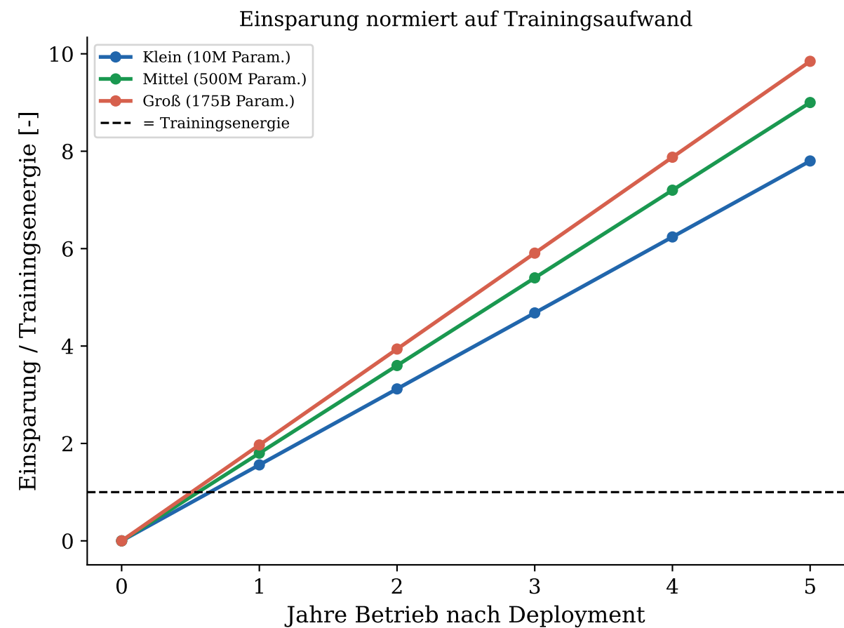
Abb. 21: Modell-Lebenszyklus-Energieanalyse: Training vs. Inferenz
