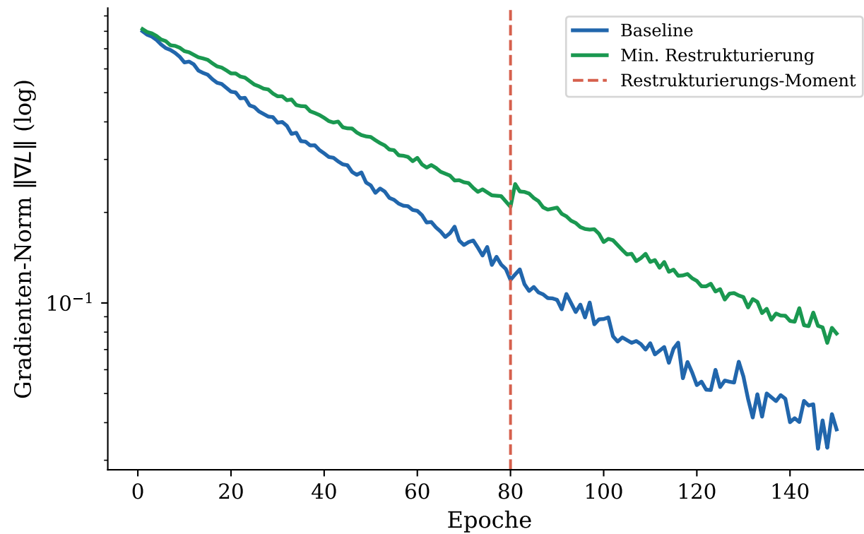
Gradienten-Norm-Verlauf
