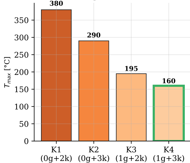
Max. Temperatur ( \downarrow =besser)
