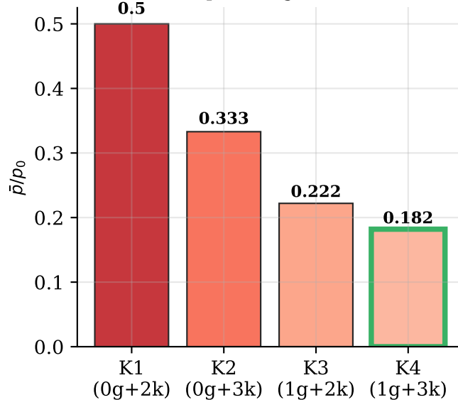
Flächenpressung ( \downarrow =besser)
