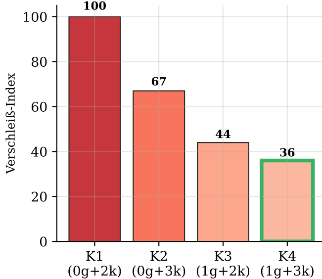
Verschleiß rel. zu K1 ( \downarrow )
