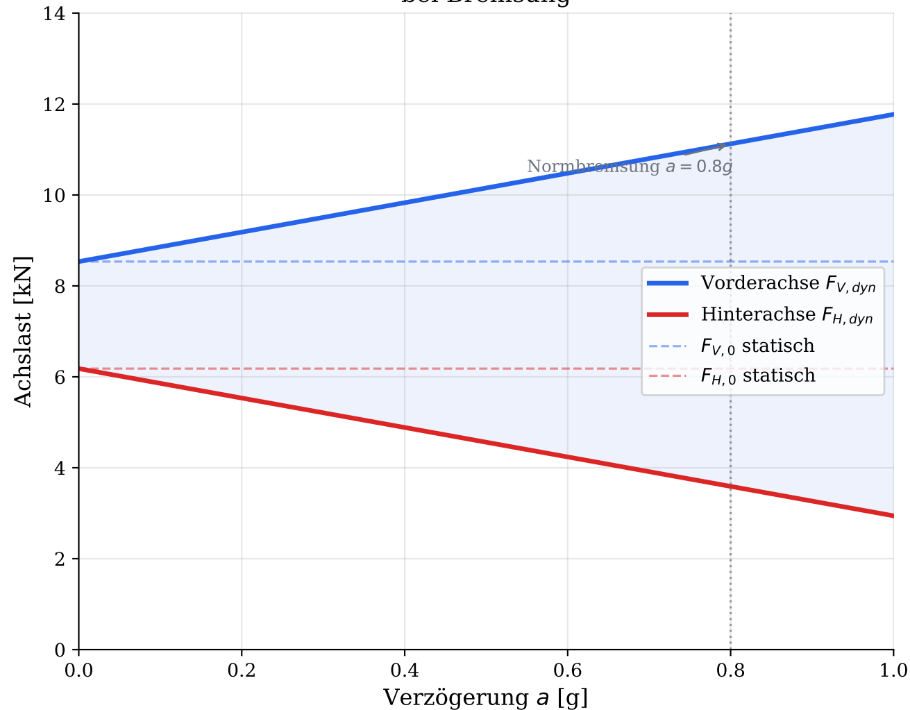
Dynamische Achslastverteilung bei Bremsung
