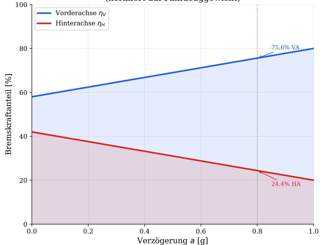
Bremskraftanteil je Achse (normiert auf Fahrzeuggewicht)
