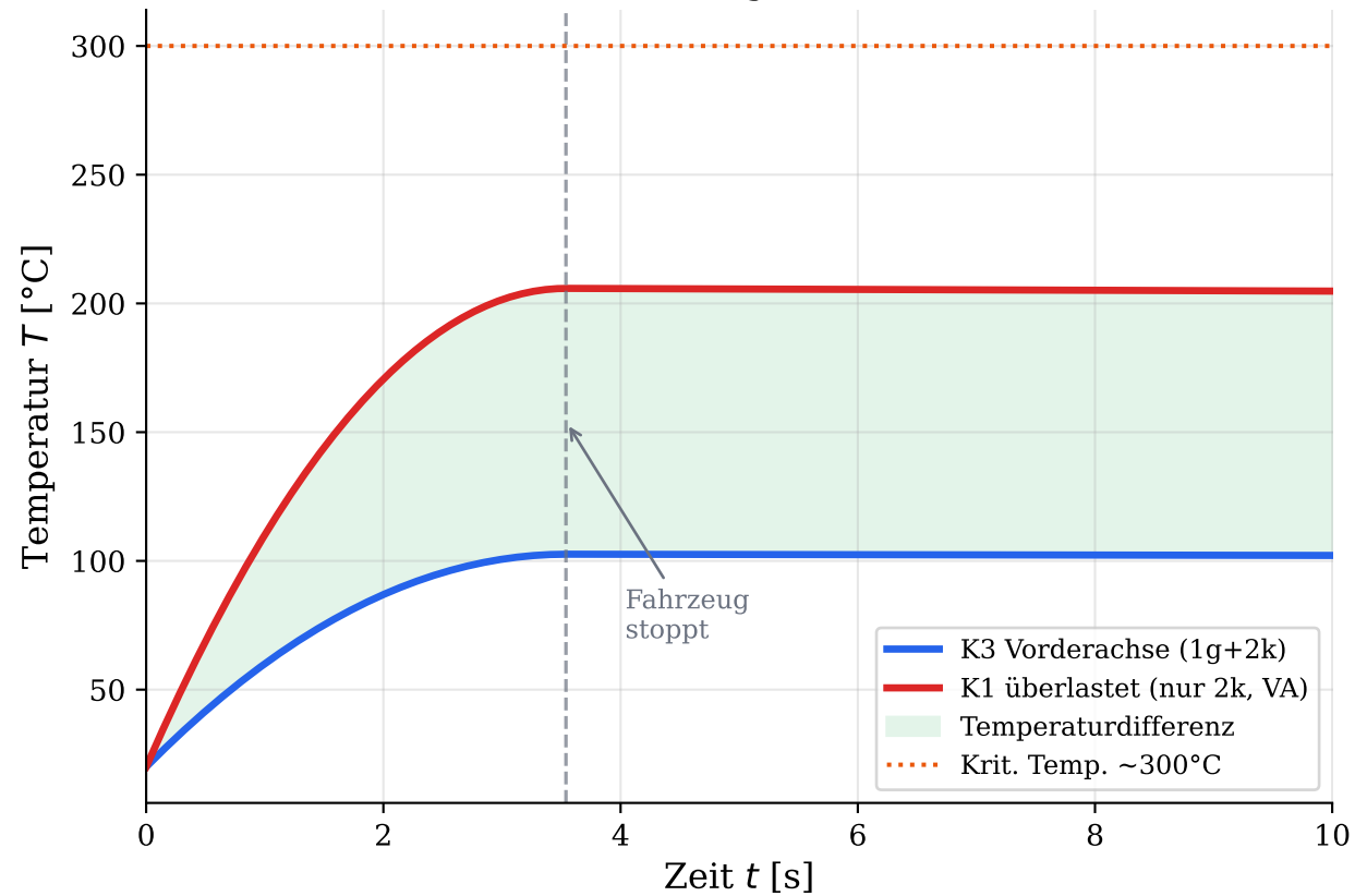
Temperaturentwicklung bei Vollbremsung (100→0 km/h)
