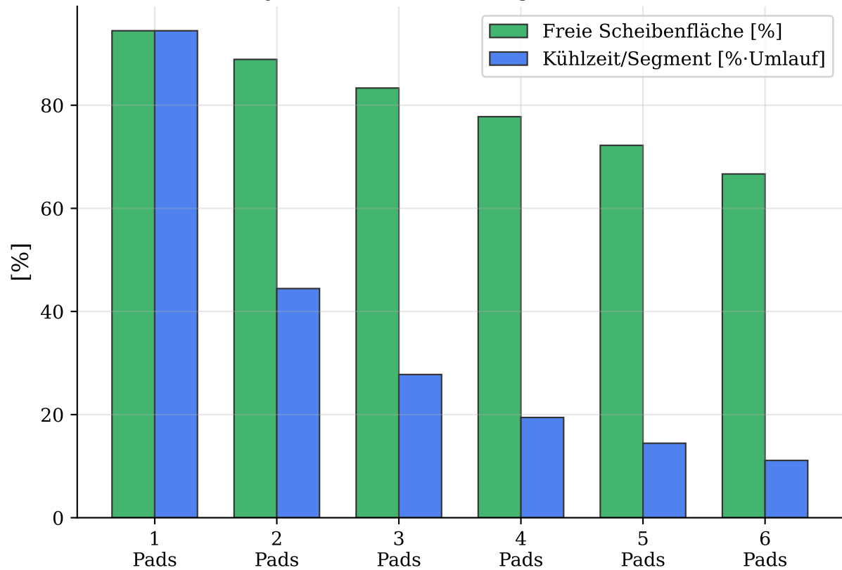
Kühlwirkung durch Segmentierung (je 20° Pad-Breite angenommen)
